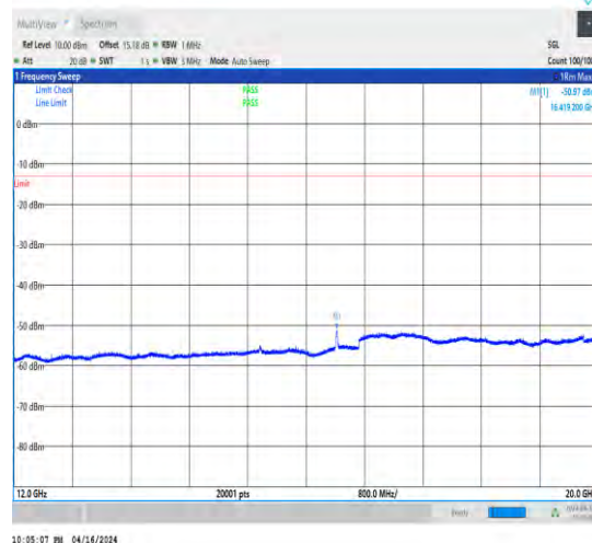
1-N5-15-20-L-1-DFT-QPSK-Edge_1RB_Left-1@0-12 000-20000-Ant1-16419.20--50.97--13-PASS
