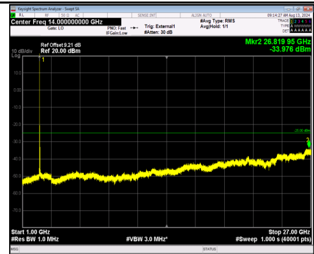
41-41-5MHz-20MHz-QPSK-QPSK-40273-40390-1RB#0-ORB#0-1000~27000MHz-PASS
