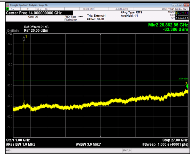
41-41-5MHz-20MHz-QPSK-QPSK-41023-41140-1RB#0-1 RB#99-1000~27000MHz-PASS
