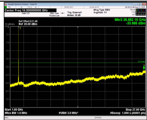
41-41-5MHz-20MHz-QPSK-QPSK-41023-41140-1RB#0-0 RB#0-1000~27000MHz-PASS
