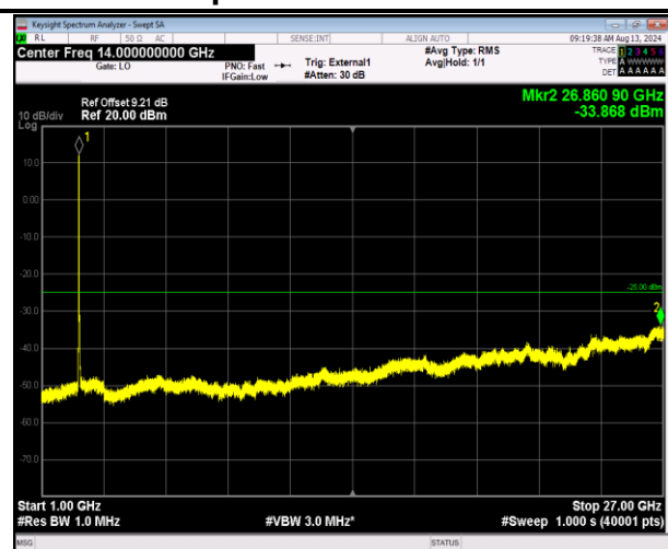
41-41-5MHz-20MHz-QPSK-QPSK-40273-40390-25RB#0- 100RB#0-1000~27000MHz-PASS
