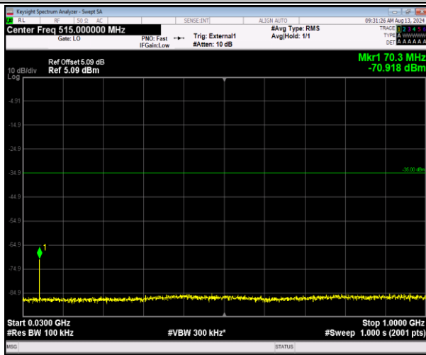
41-41-5MHz-20MHz-QPSK-QPSK-41023-41140-1RB#0- 1RB#99-30~1000MHz-PASS
