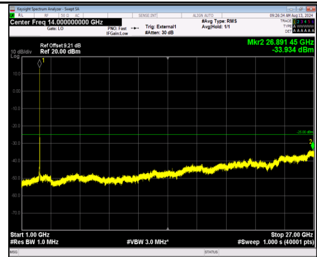
41-41-5MHz-20MHz-QPSK-QPSK-40648-40765-25RB#0- 100RB#0-1000~27000MHz-PASS
