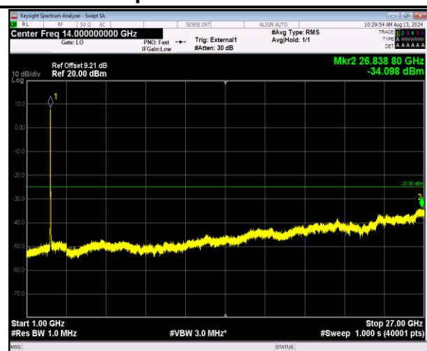
41-41-20MHz-5MHz-QPSK-QPSK-40340-40457-100RB# 0-25RB#0-1000~27000MHz-PASS
