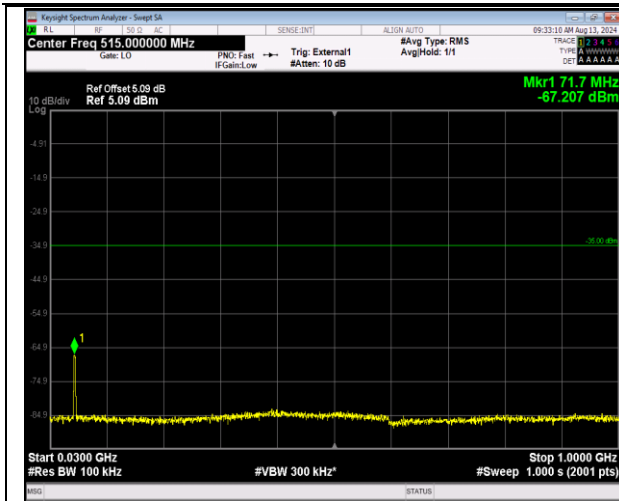
41-41-5MHz-20MHz-QPSK-QPSK-41023-41140-25RB#0 -100RB#0-30~1000MHz-PASS
