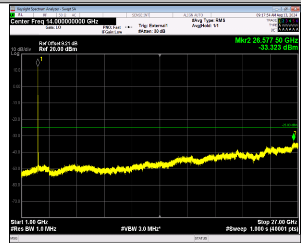
41-41-5MHz-20MHz-QPSK-QPSK-40273-40390-1RB#0-1RB#99-1000~27000MHz-PASS
