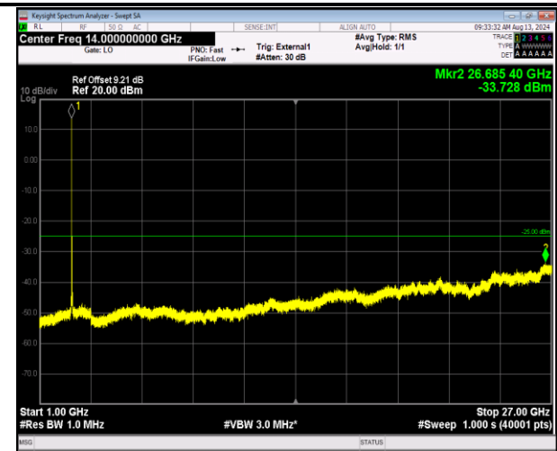
41-41-5MHz-20MHz-QPSK-QPSK-41023-41140-25RB#0- 100RB#0-1000~27000MHz-PASS
