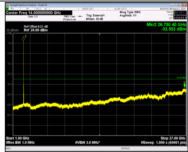
41-41-5MHz-20MHz-QPSK-QPSK-40648-40765-1RB#0-1RB#99-1000~27000MHz-PASS
