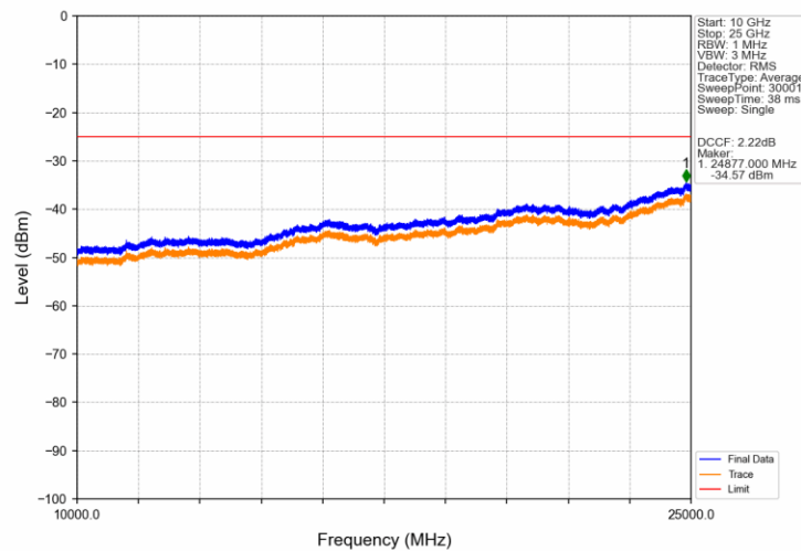
Band41 5MHz 16QAM LCH 2557.5MHz RB 1 0 NTNV
