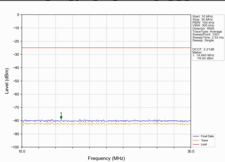
Band41_5MHz_QPSK_HCH_2652.5MHz_RB_1_0_NTNV
