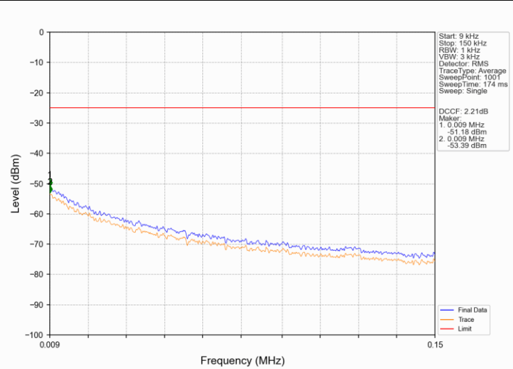
Band41_5MHz_QPSK_MCH_2605MHz_RB_1_0_NTNV
