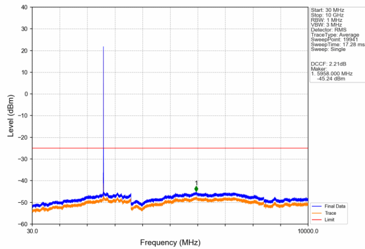
Band41_5MHz_QPSK_MCH_2605MHz_RB_1_0_NTNV
