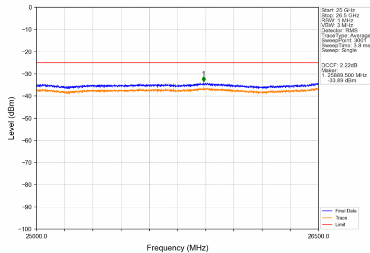
Band41 5MHz 16QAM MCH 2605MHz RB 1 0 NTV
