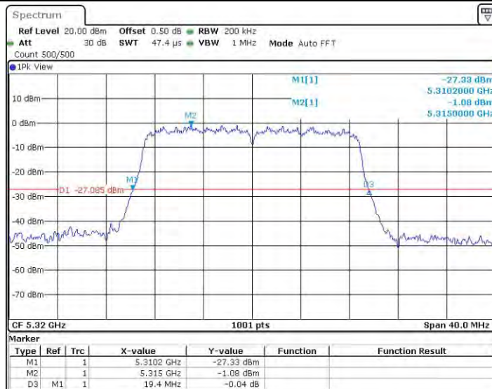
11N20MIMO_Ant0_5320
