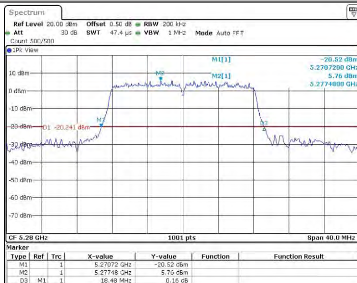
11A_Ant0_5280
