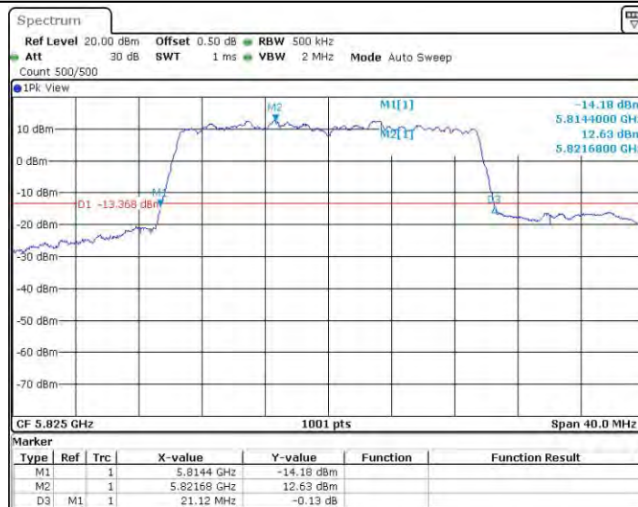
11AX20SISO_Ant0_5825
