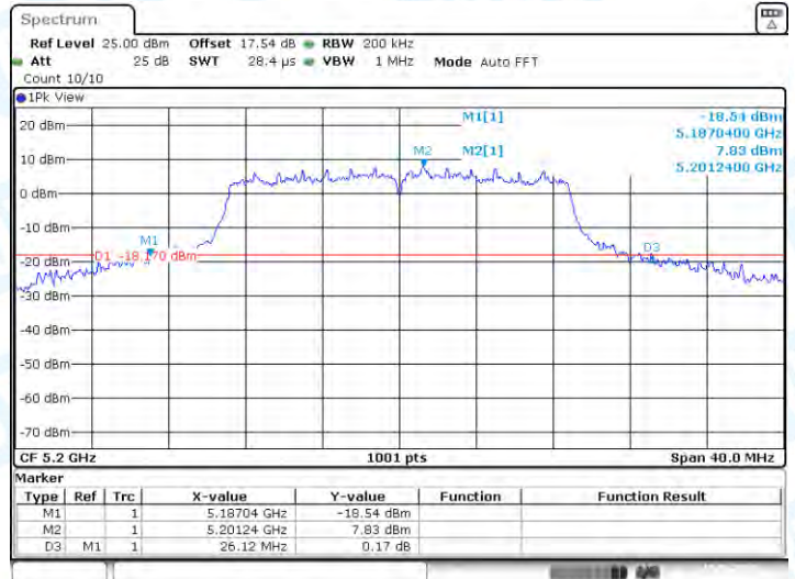
11N20-CDD-Ant1-5200
