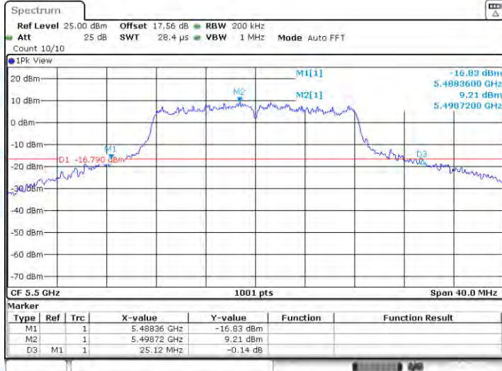
11A-Ant1-5500
