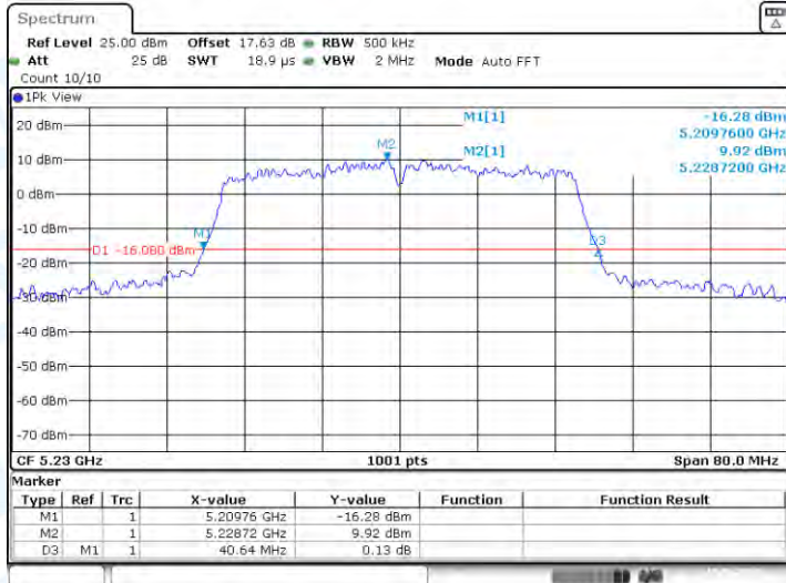
11N40-CDD-Ant1-5230
