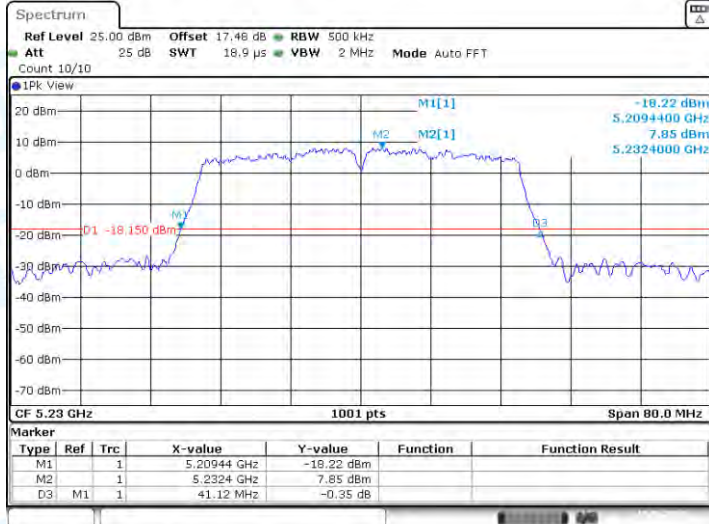
11N40-CDD-Ant1-5230
