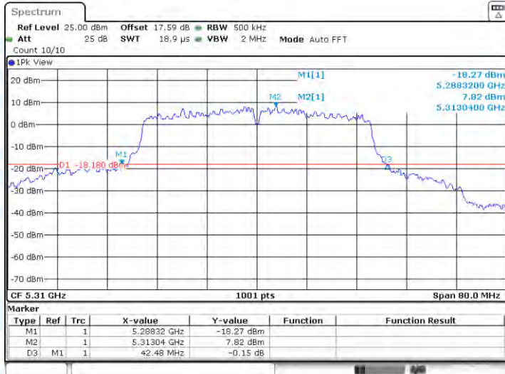
11N40-CDD-Ant1-5310
