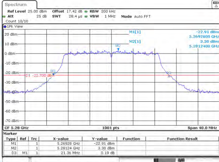
11N20-CDD-Ant1-5280
