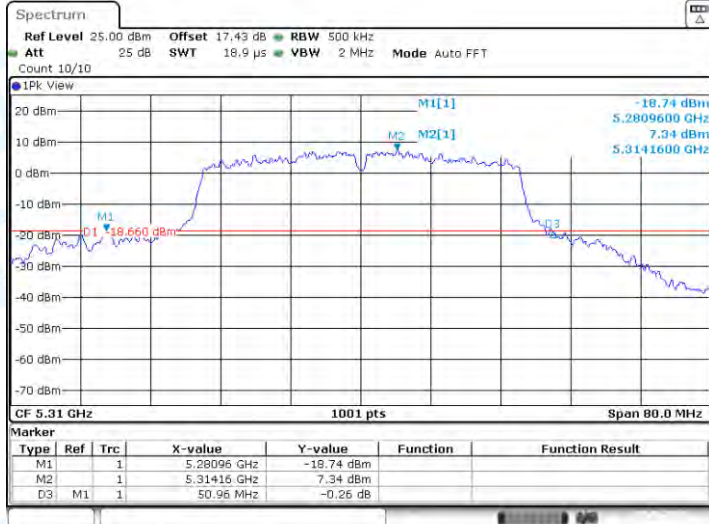
11N40-CDD-Ant1-5310
