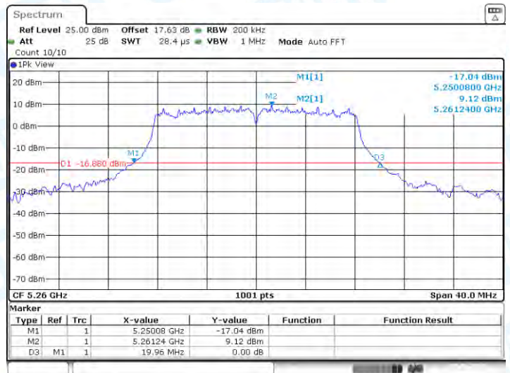
11A-Ant1-5260
