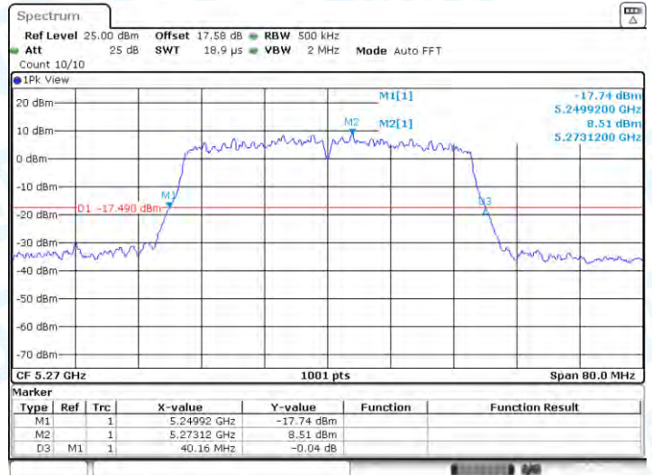
11N40-CDD-Ant1-5270
