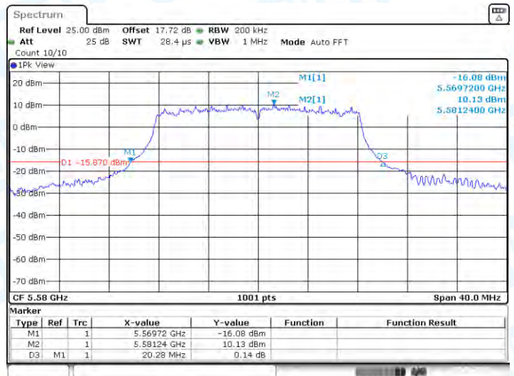
11A-Ant1-5580
