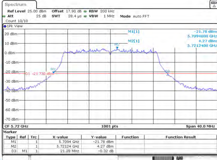
11N20-CDD-Ant1-5720
