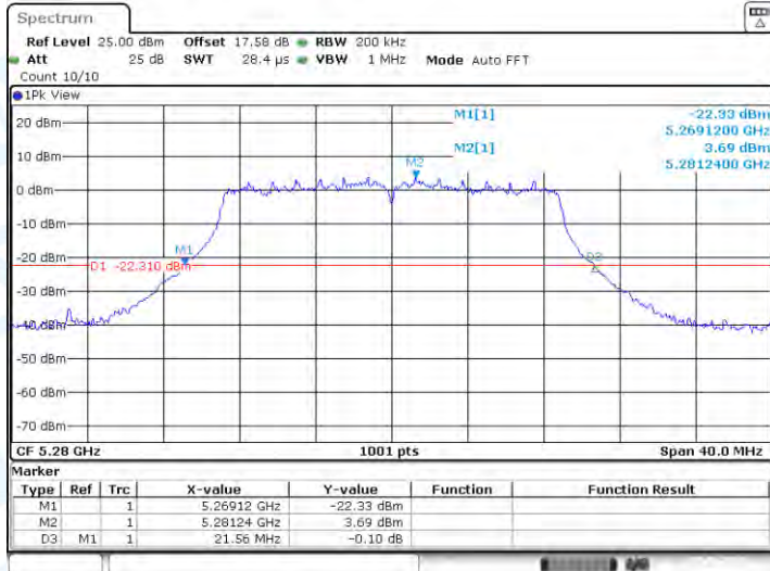
11N20-CDD-Ant1-5280
