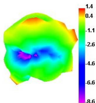
2450.000MHz E1
