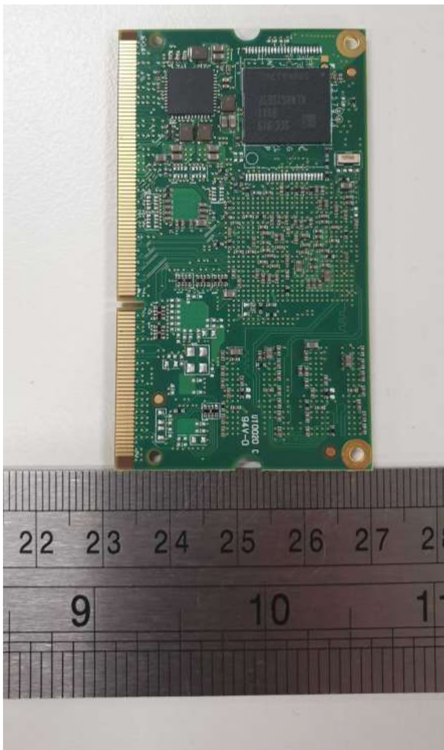
Module Back
