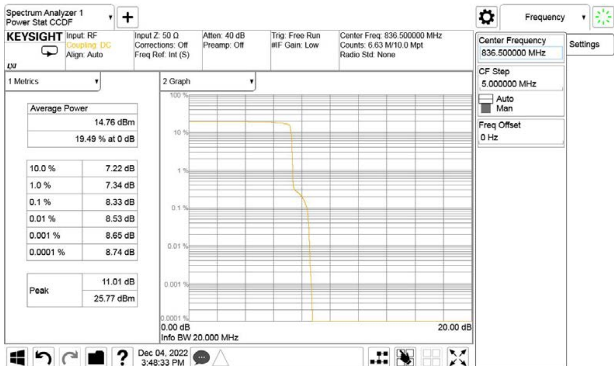
Band26-CH26915-836.5MHz-BPSK
