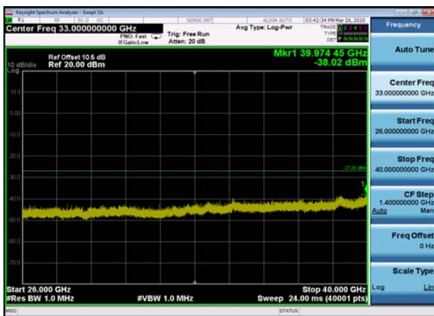
U-NII-1 ,Plot 4,26000MHz~40000MHz-802 .11ac(20MHz),5180MHz,Ant1
