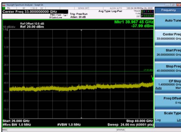
U-NII-1 ,Plot 4,26000MHz~40000MHz-802 .11ac(40MHz),5230MHz,Ant1
