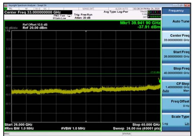
U-NII-1 ,Plot 4,26000MHz~40000MHz-802 .11ac(20MHz),5220MHz,Ant1
