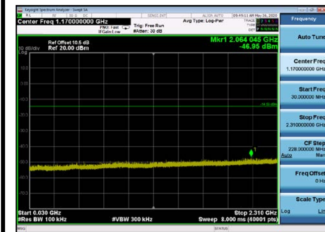
,Plot 3,30MHz~2310MHz-802.11g,2437MHz
