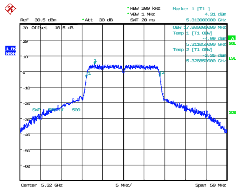
802.11n20_5320MHz
