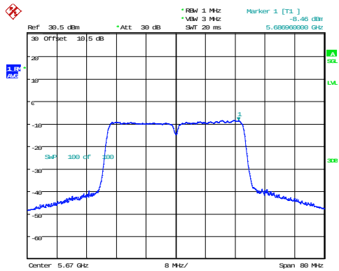
802.11ac40_5670MHz
