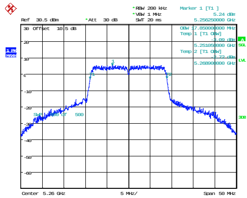
802.11n20_5260MHz
