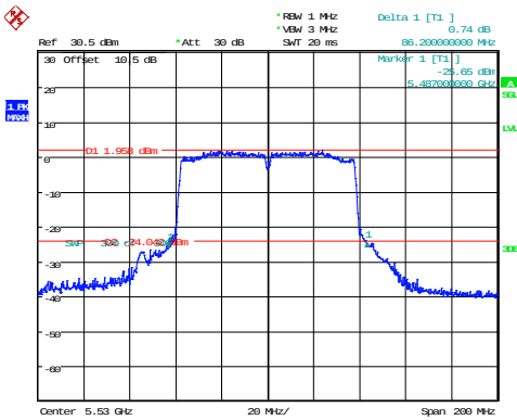
802.11ac80_5530MHz
