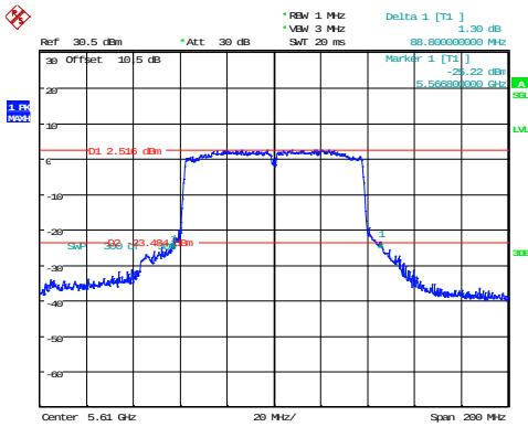
802.11ac80_5610MHz
