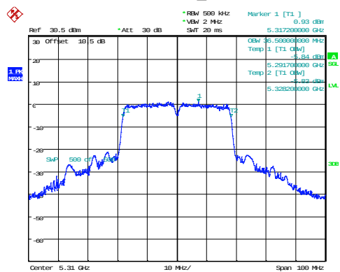
802.11ac40_5310MHz
