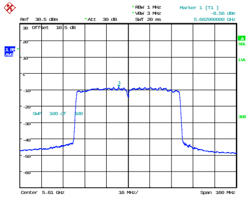
802.11ac80_5610MHz
