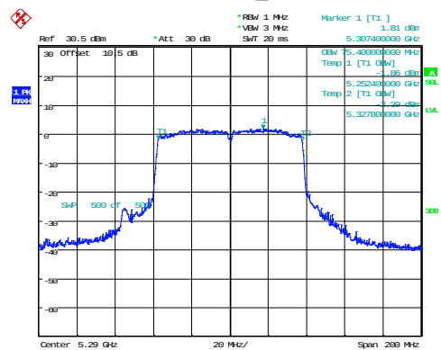
802.11ac80_5290MHz
