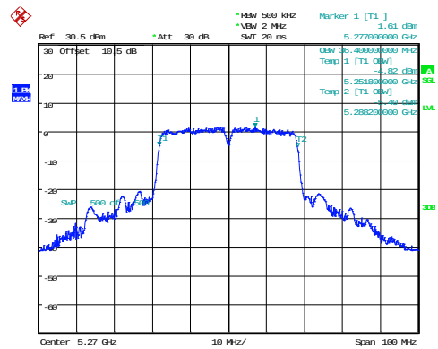
802.11ac40_5270MHz
