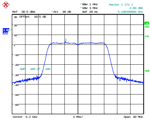
802.11n20_5200MHz
