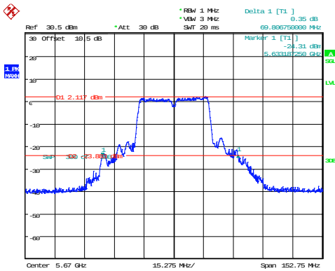
802.11ac40_5670MHz
