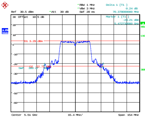
802.11ac40_5510MHz
