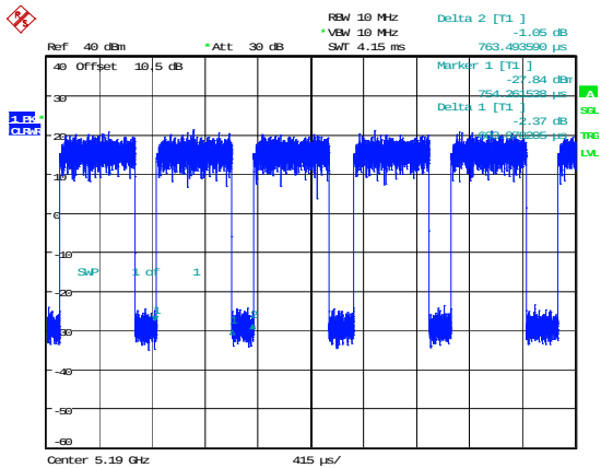
802.11ac40_5190MHz
