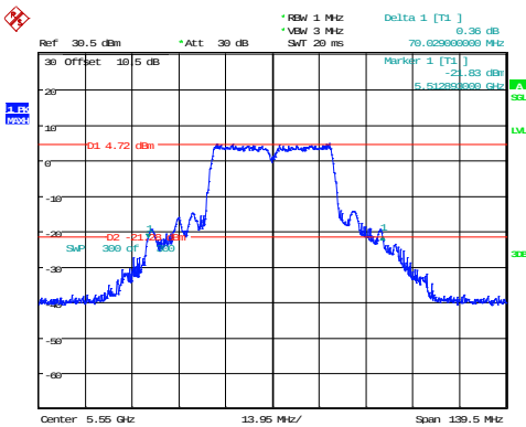
802.11ac40_5550MHz
