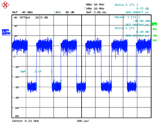
802.11ac80_5210MHz
