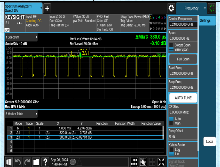
NTNV-11AC80SISO-Ant2-5210
