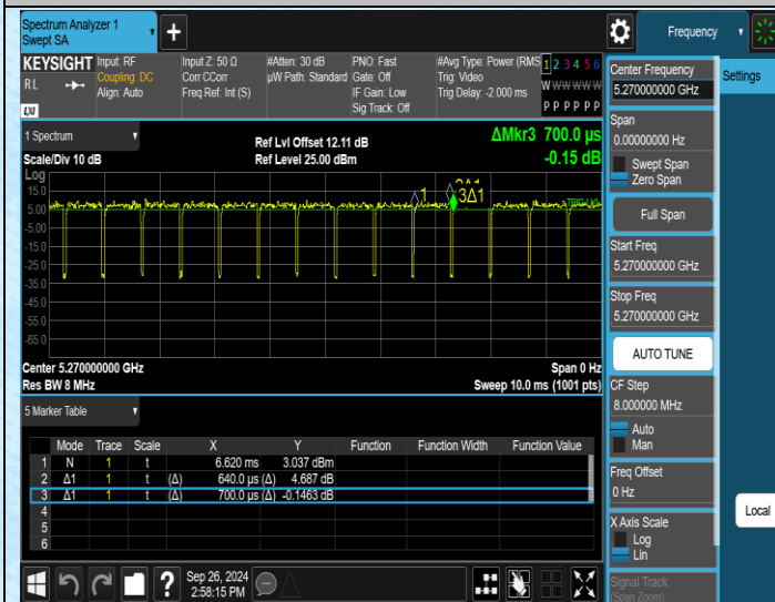
NTNV-11N40MIMO-Ant1-5270
