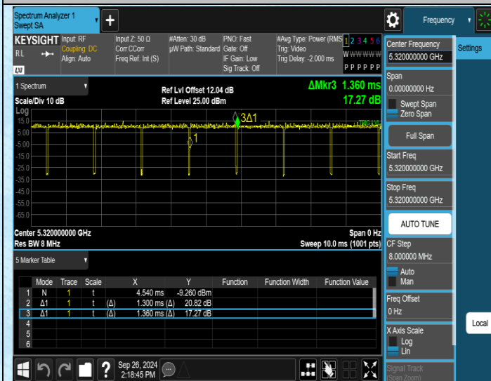
NTNV-11N20MIMO-Ant1-5320
