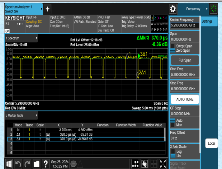
NTNV-11AC80SISO-Ant2-5290
