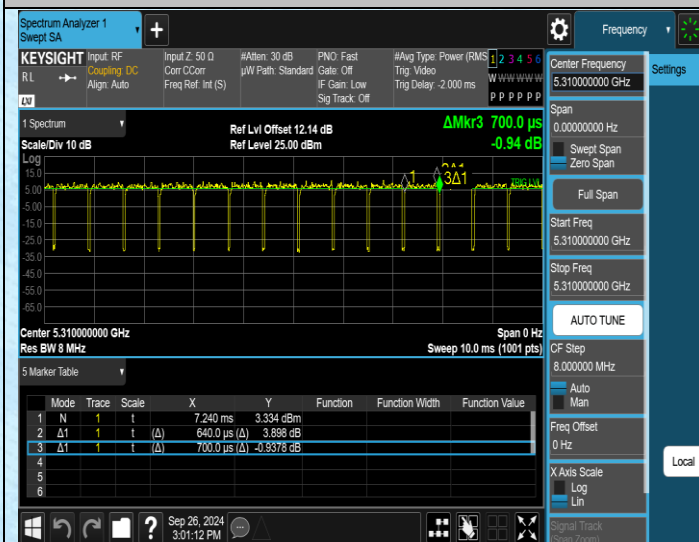
NTNV-11N40MIMO-Ant1-5310
