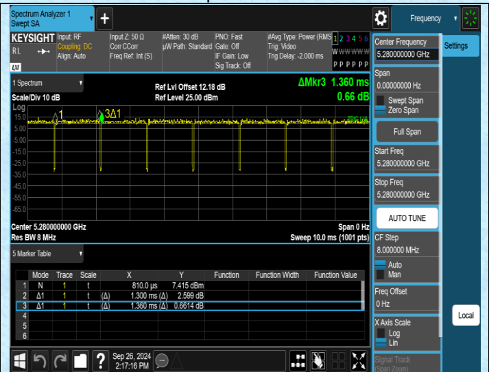
NTNV-11N20MIMO-Ant2-5280
