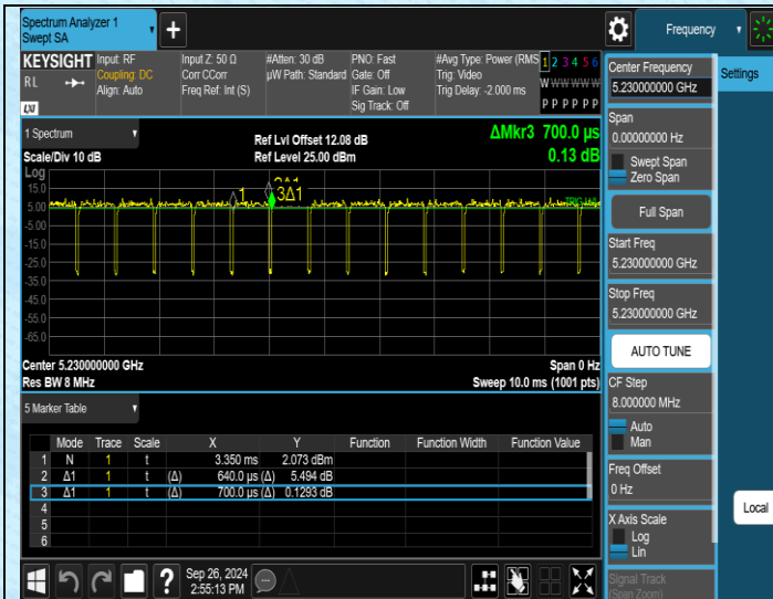
NTNV-11N40MIMO-Ant1-5230
