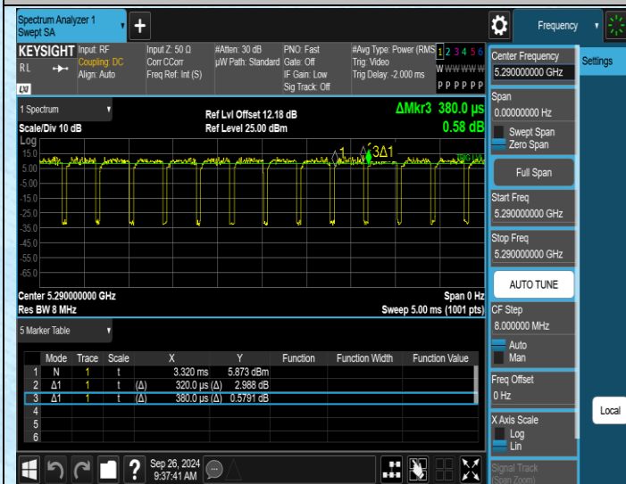
NTNV-11AC80SISO-Ant1-5290
