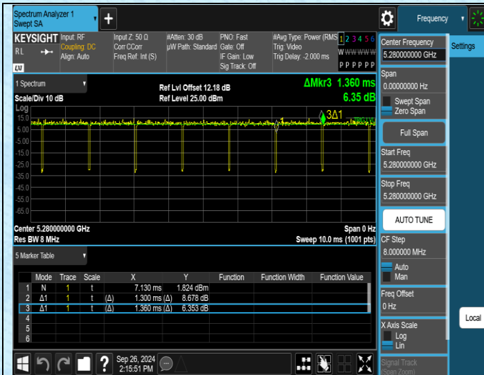
NTNV-11N20MIMO-Ant1-5280
