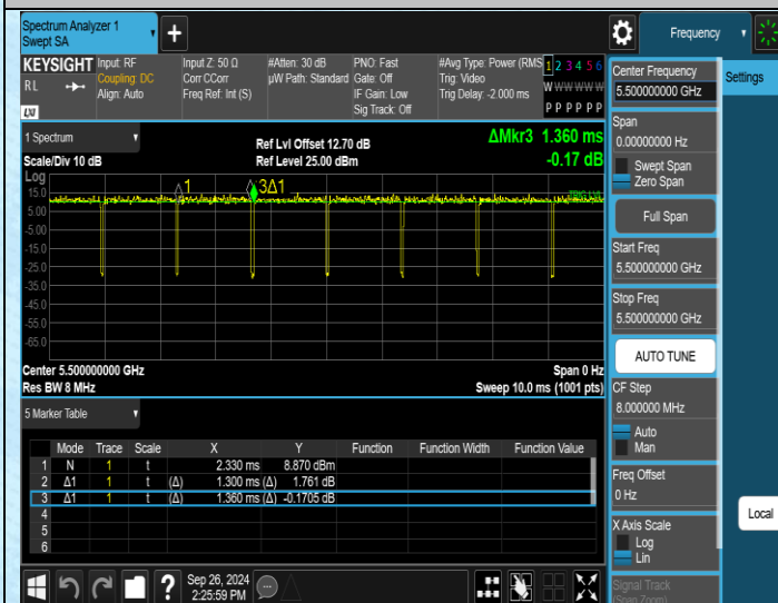
NTNV-11N20MIMO-Ant1-5500
