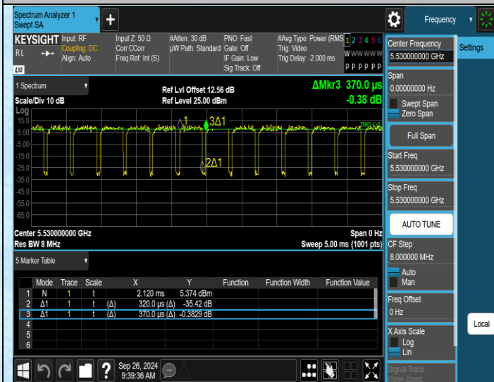
NTNV-11AC80SISO-Ant1-5530
