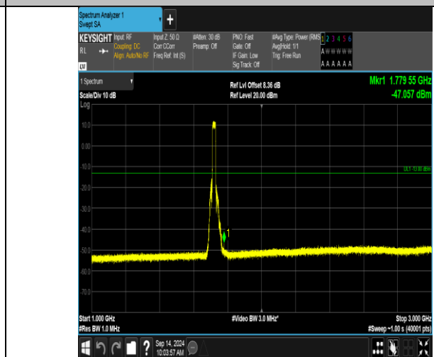
Band66_20MHz_QPSK_132072_100RB#0_1000~3000_1000~3000
