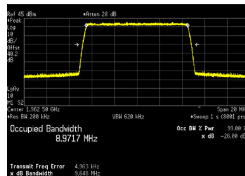
LTE10_64QAM
