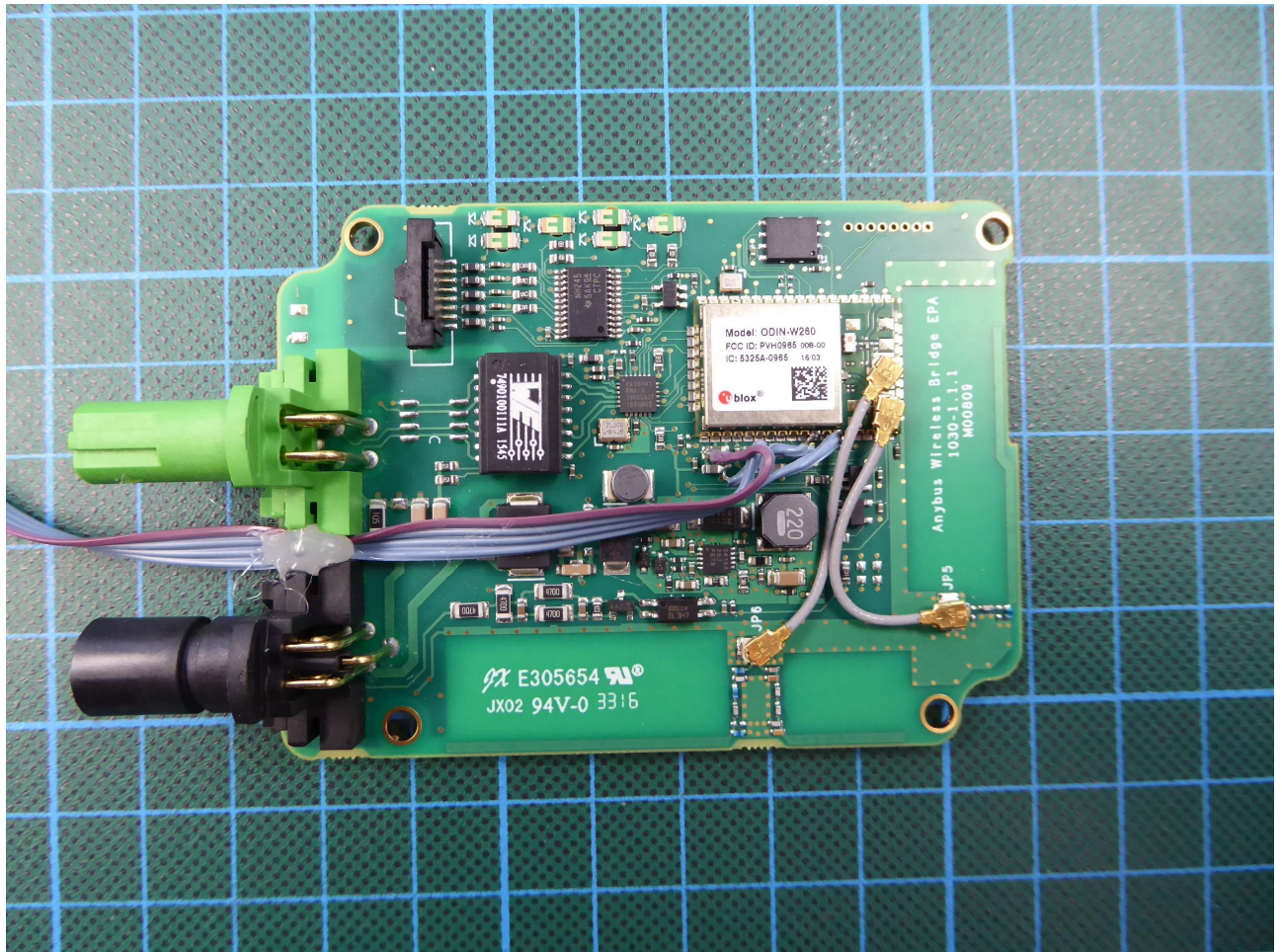
161944eut002: EUT Detail top view
