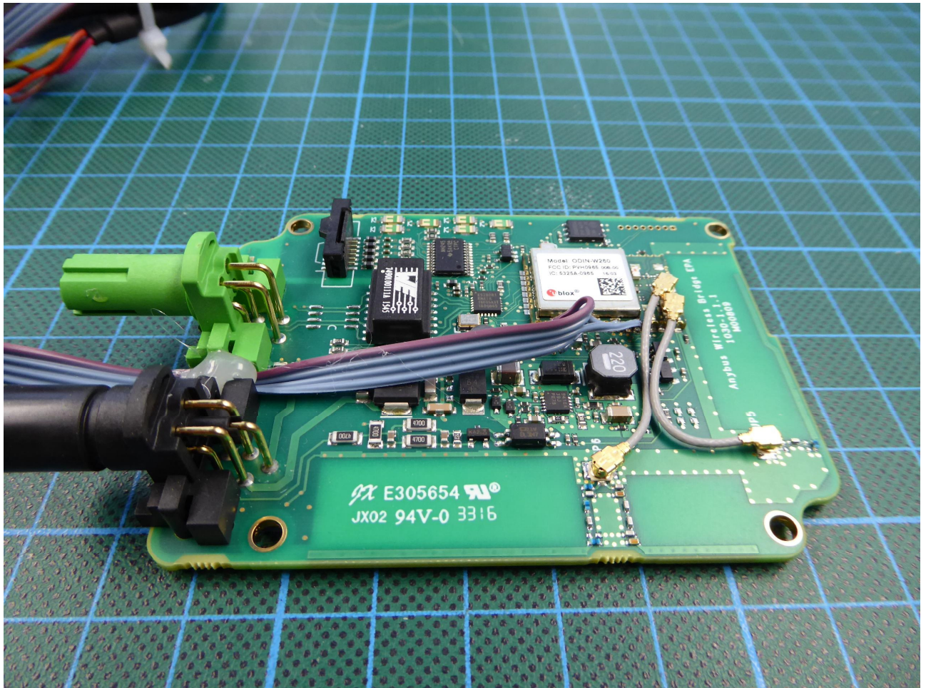
161944eut003: EUT side view
