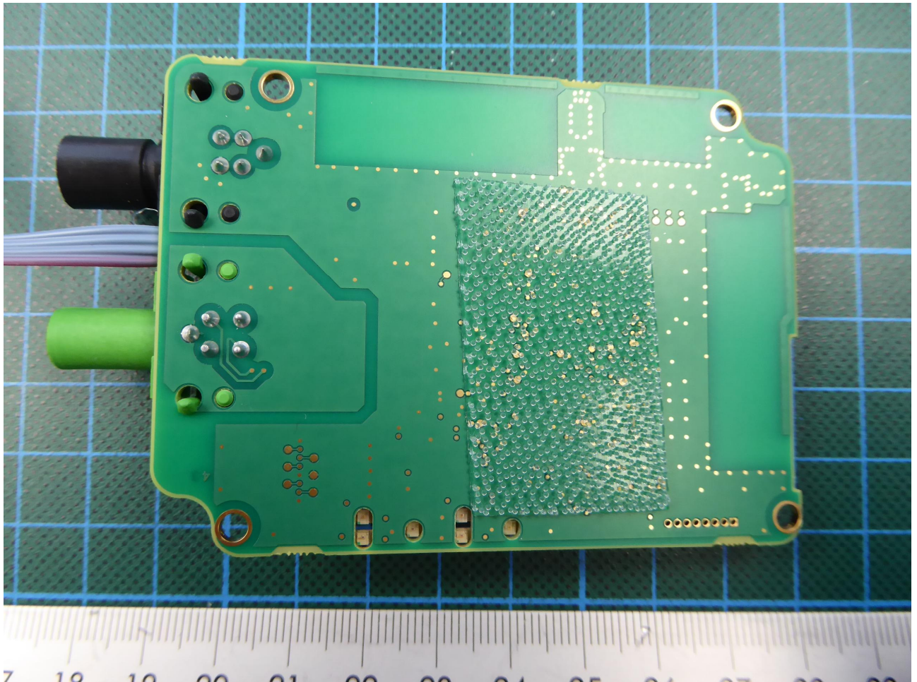
161944eut005:EUT back view
