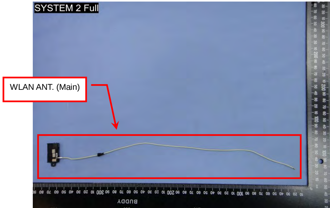
EUT Photo (24)
