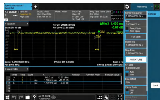
NTVN-11AX80SISO-Ant1-5530-484Tone-RU65
