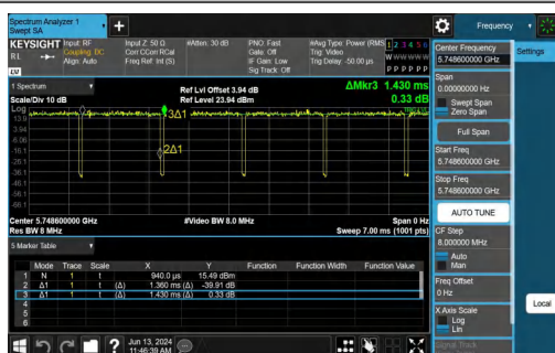
NTVN-11AX80SISO-Ant1-5775-484Tone-RU65
