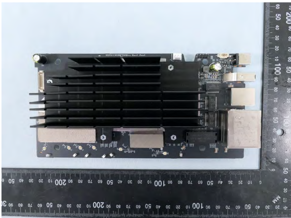
(40) EUT Photo – Archer BE700 Pro
