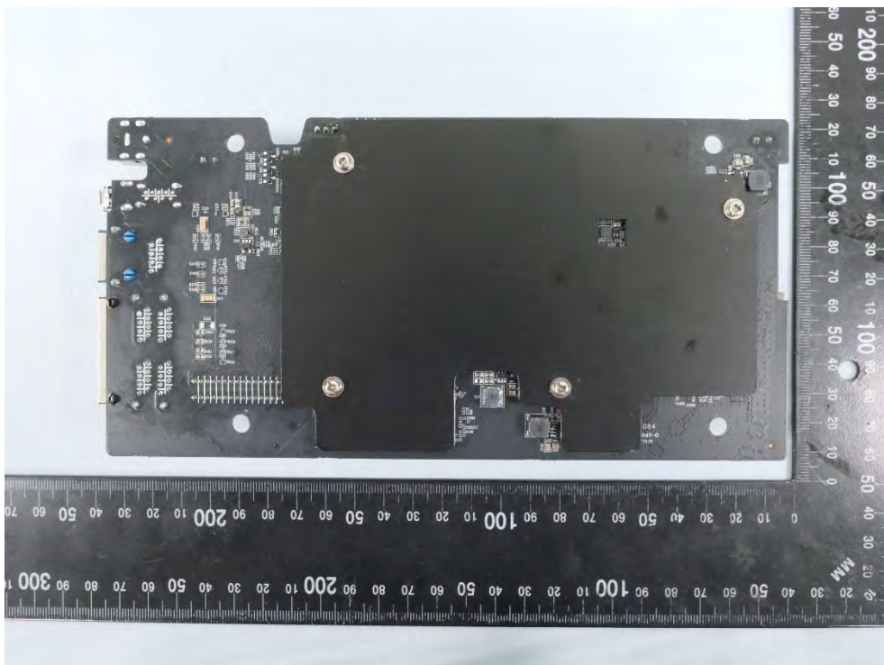
(22) EUT Photo – Archer BE700
