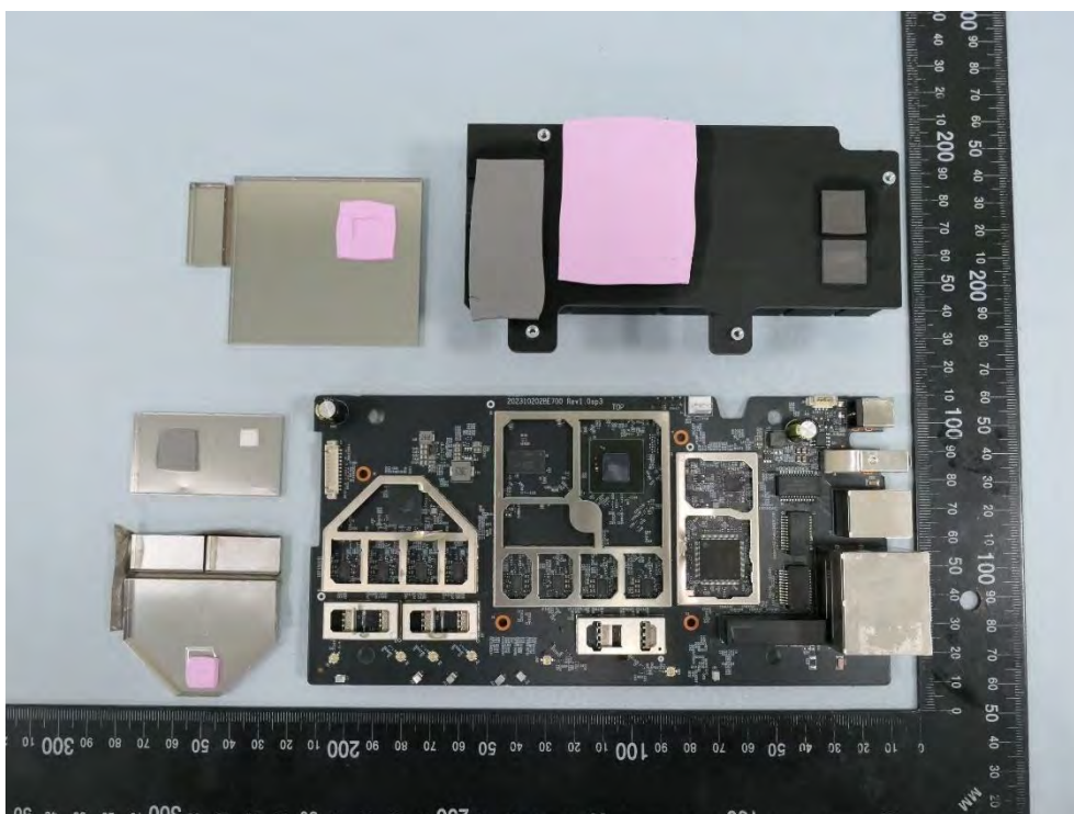
(12) EUT Photo – Archer BE700
