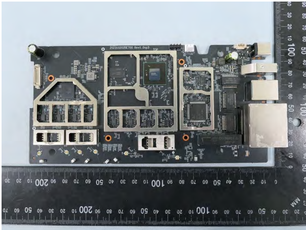
(14) EUT Photo – Archer BE700
