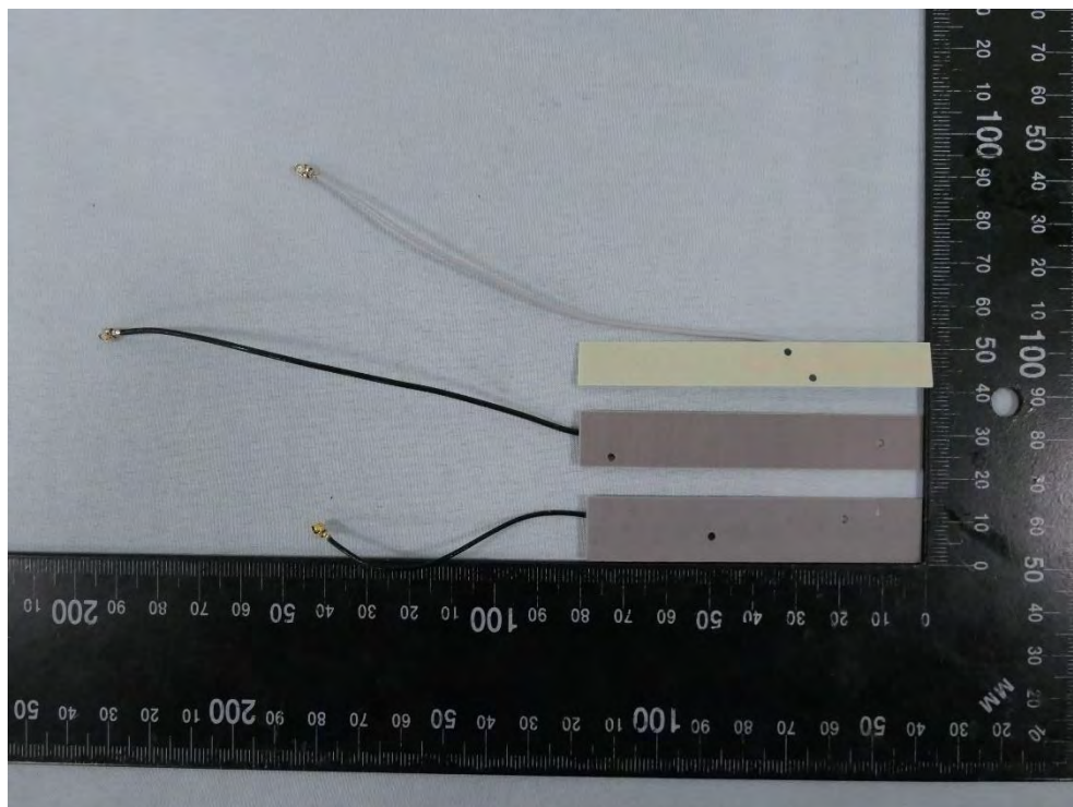
(10) EUT Photo – Archer BE700
