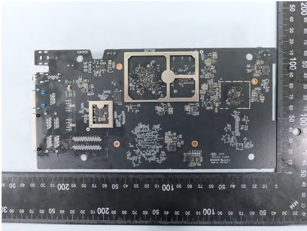
(54) EUT Photo – Archer BE700 Pro
