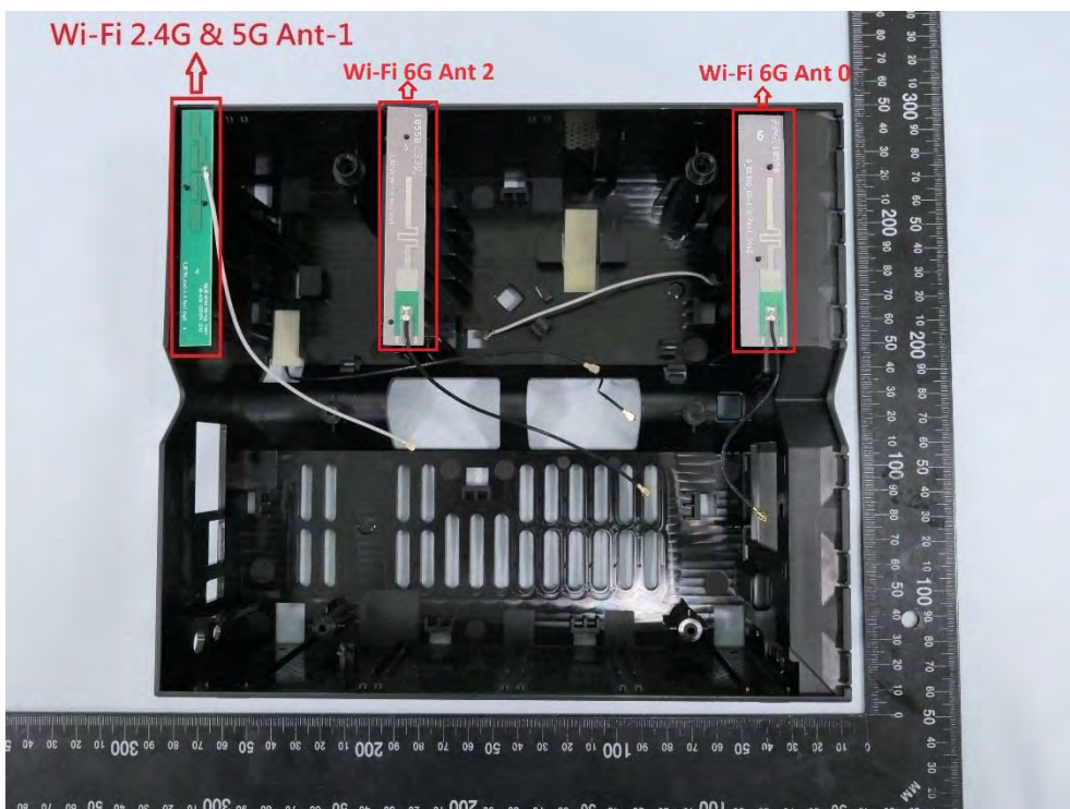
(4) EUT Photo – Archer BE700
