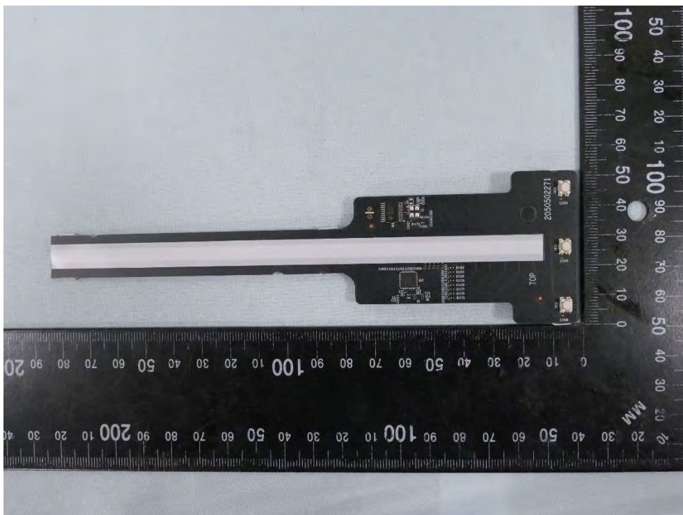
(56) EUT Photo – Archer BE700 Pro
