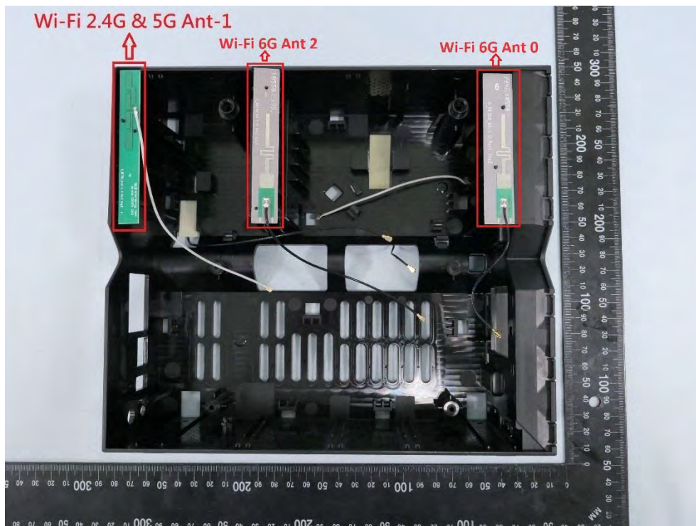
(34) EUT Photo – Archer BE700 Pro
