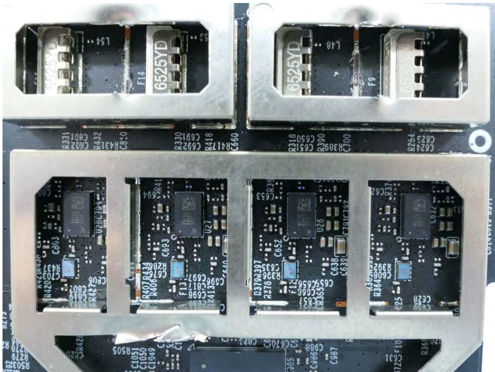
(20) EUT Photo – Archer BE700
