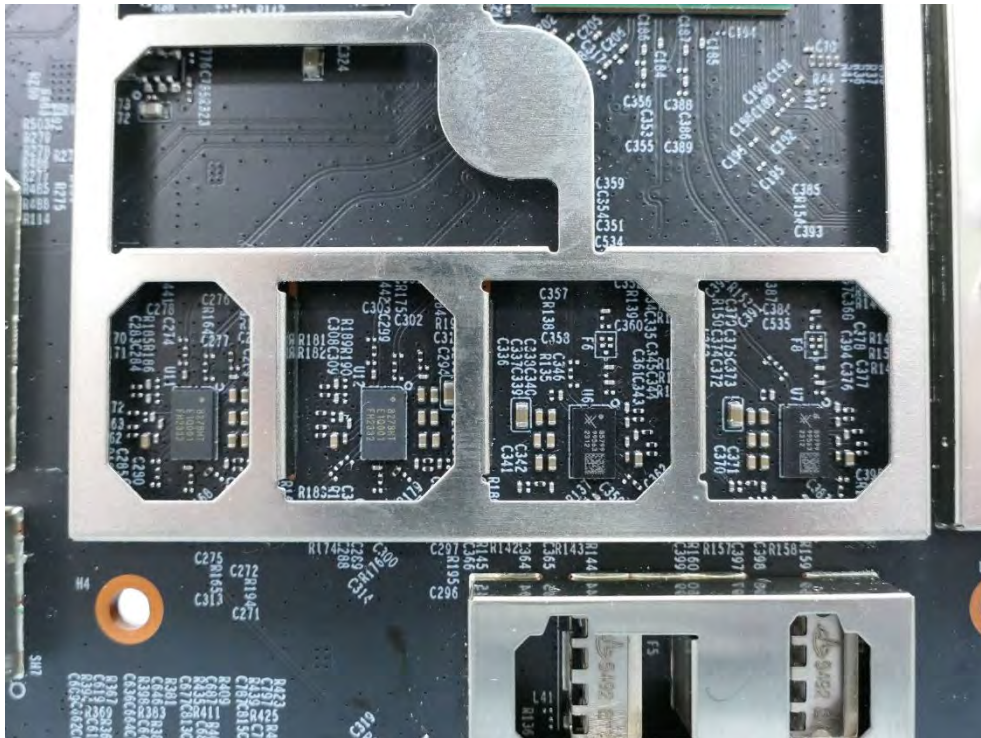
(18) EUT Photo – Archer BE700
