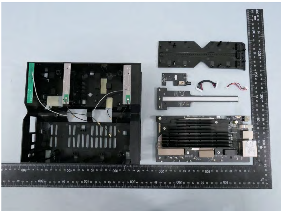
(32) EUT Photo – Archer BE700 Pro
