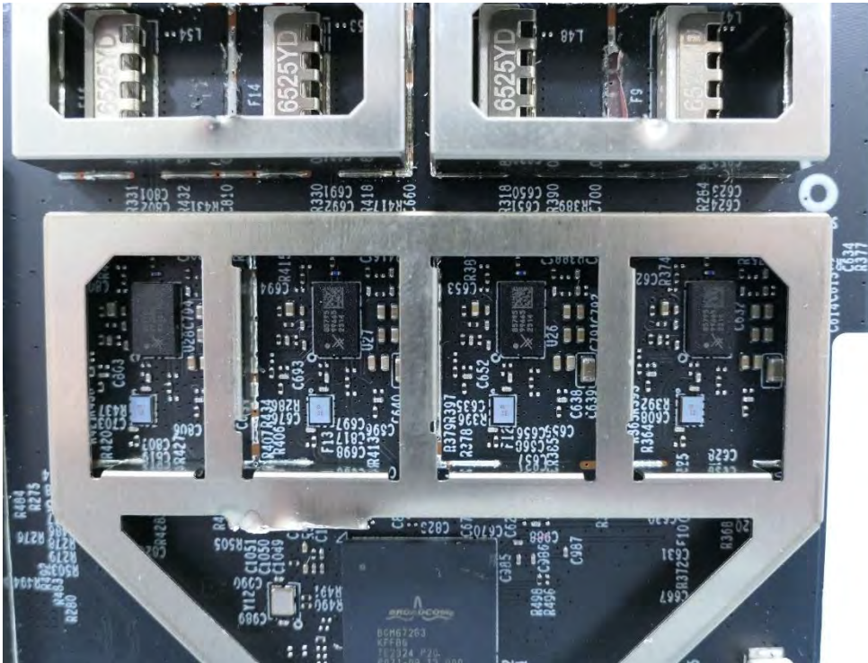
(50) EUT Photo – Archer BE700 Pro
