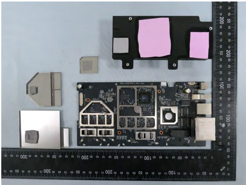
(42) EUT Photo – Archer BE700 Pro
