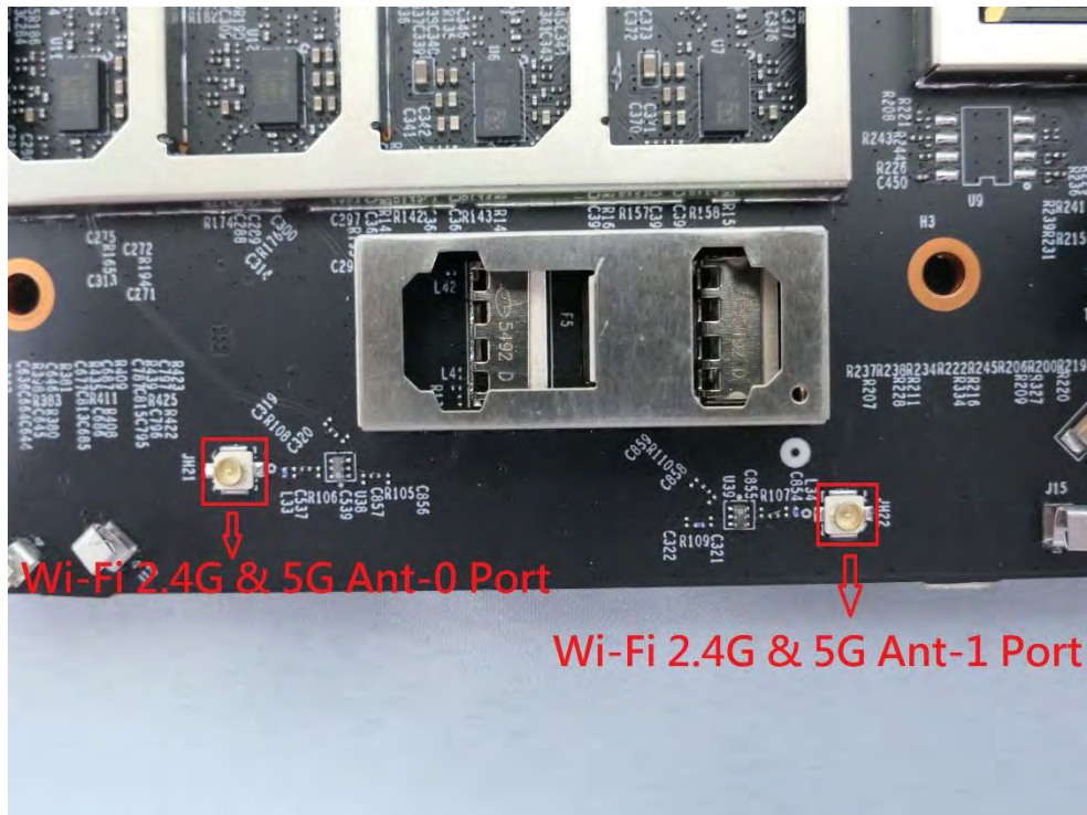
(48) EUT Photo – Archer BE700 Pro
