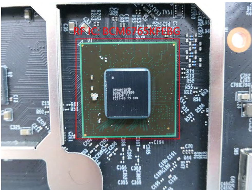
(44) EUT Photo – Archer BE700 Pro
