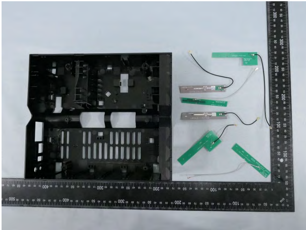
(36) EUT Photo – Archer BE700 Pro
