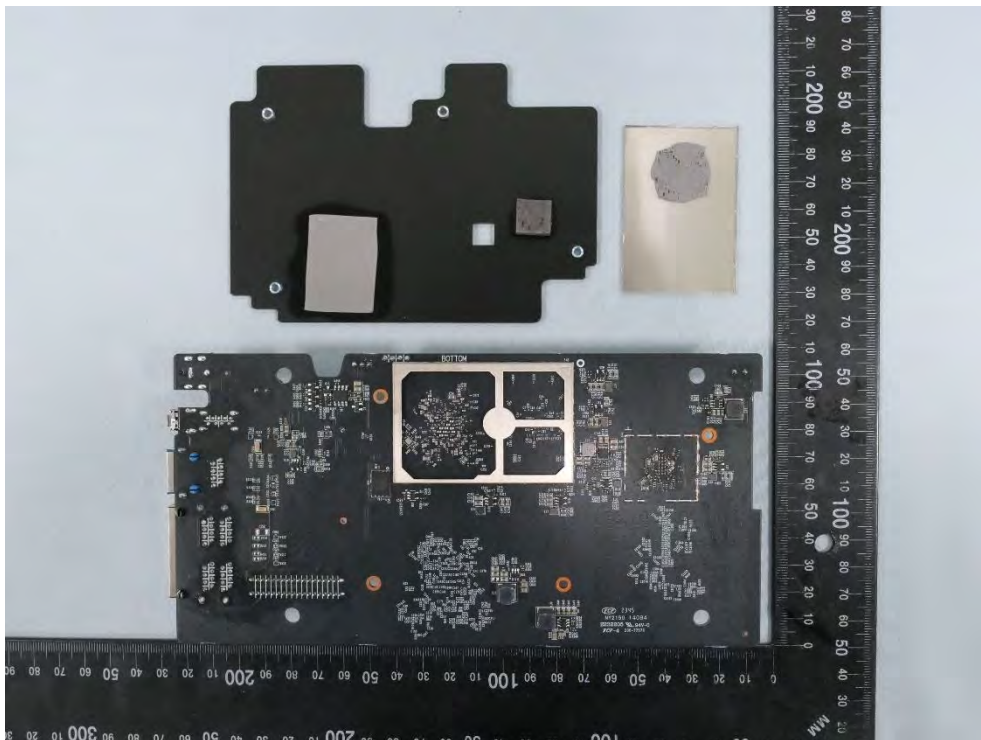
(24) EUT Photo – Archer BE700
