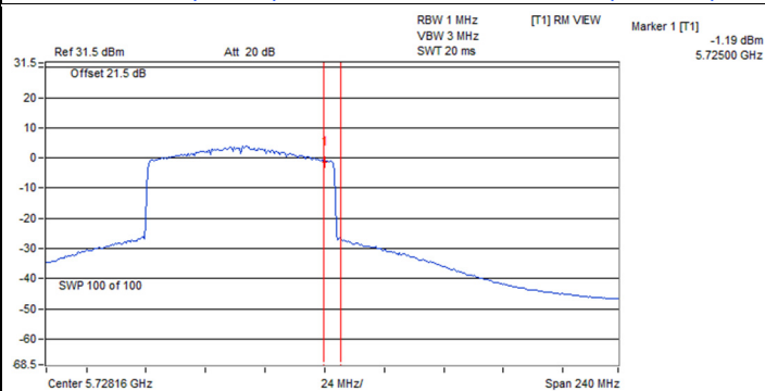
802.11ax (HE40) CDD / Chain 1 : CH 142 (U-NII-3)
