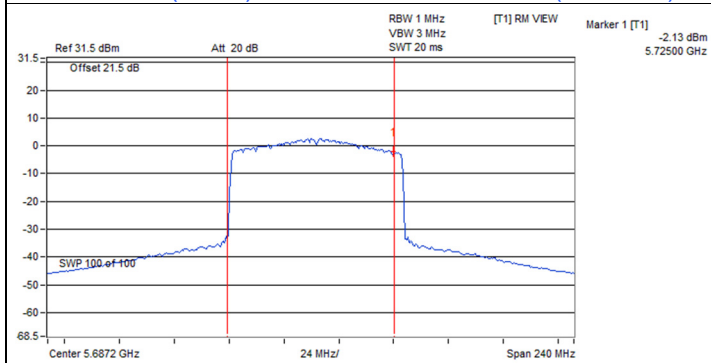
802.11ax (HE80) CDD / Chain 0 : CH 138 (U-NII-2C)
