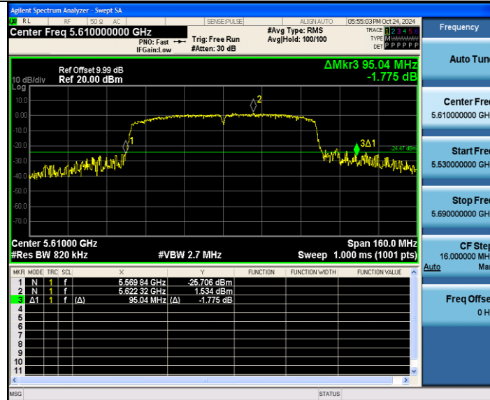
11AC80MIMO_Ant2_5610
