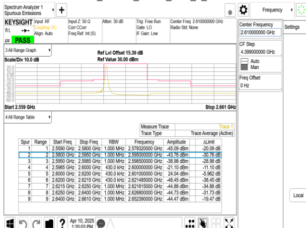
Band38_20MHz_QPSK_RB1_99_CH38150
