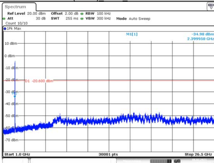
802.11n(HT20) 2412_1000~26500
