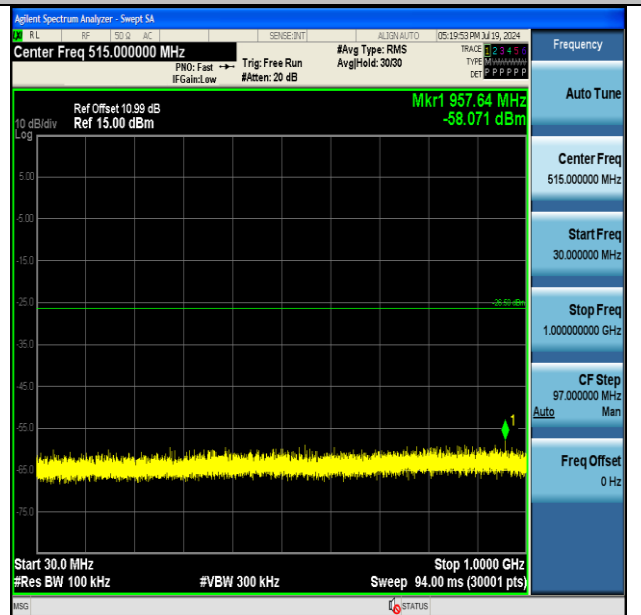
11G-Ant1-2437-30~1000-PASS
