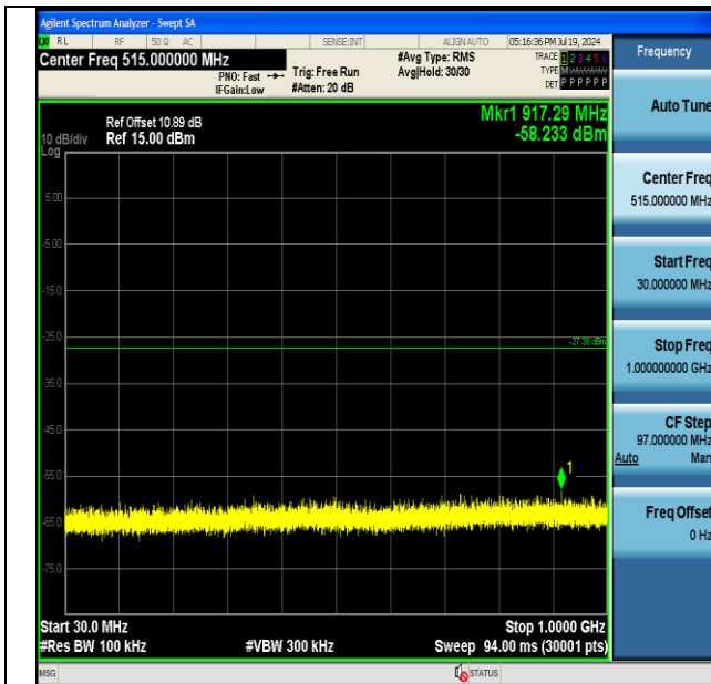
11G-Ant1-2412-30~1000-PASS
