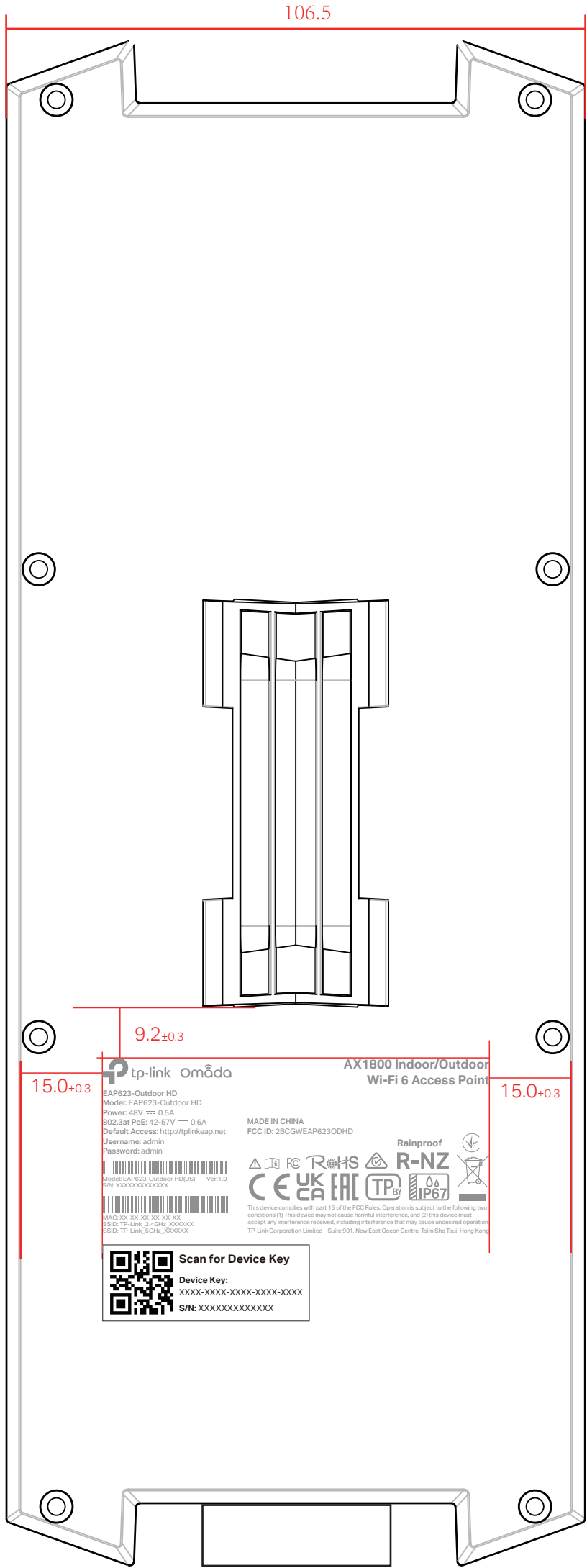
尺寸图
