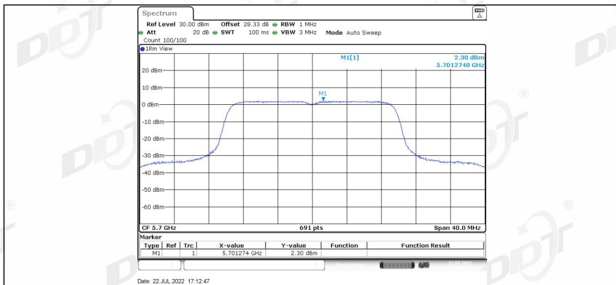
11AX20MIMO_Ant2_5700
