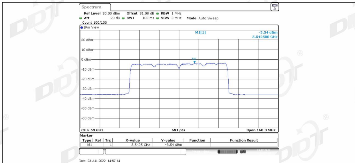
11AX80MIMO_Ant2_5530
