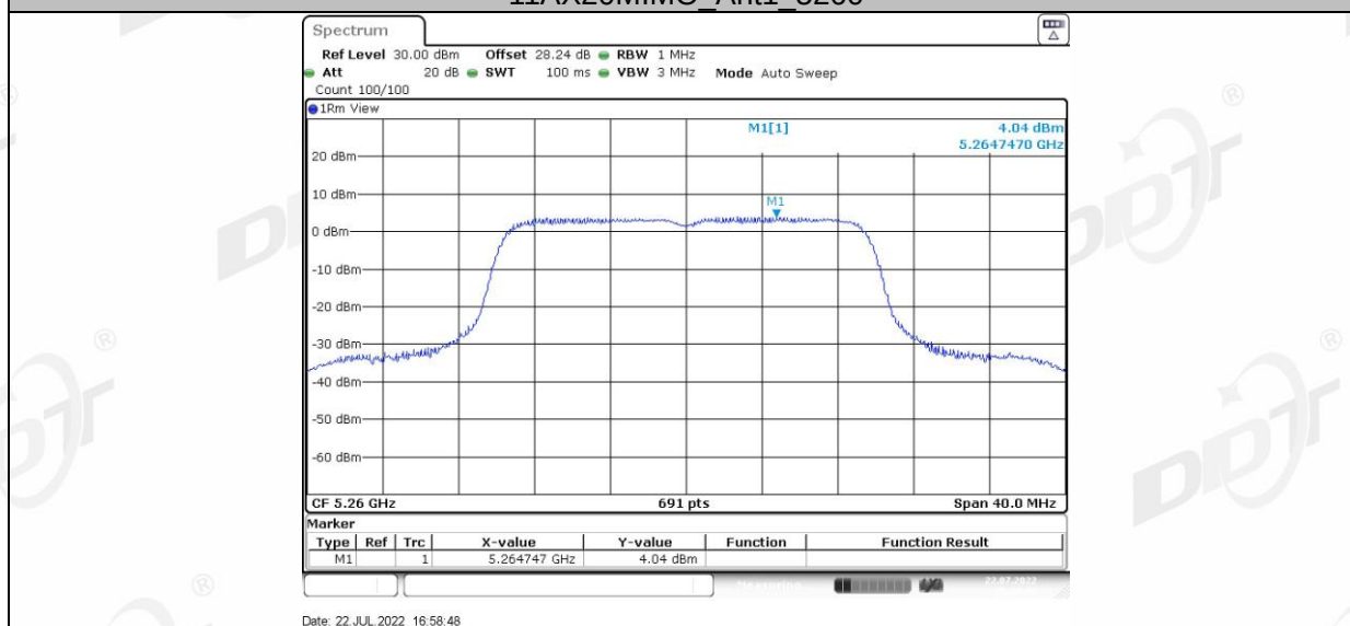
11AX20MIMO_Ant2_5260
