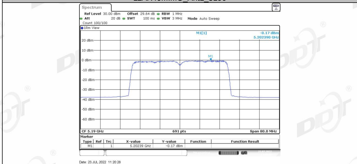
11AX40MIMO_Ant2_5190
