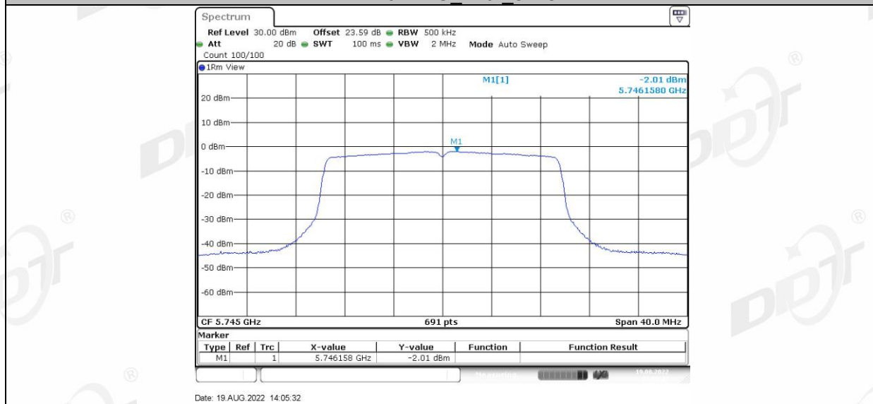
11AX20MIMO_Ant2_5745
