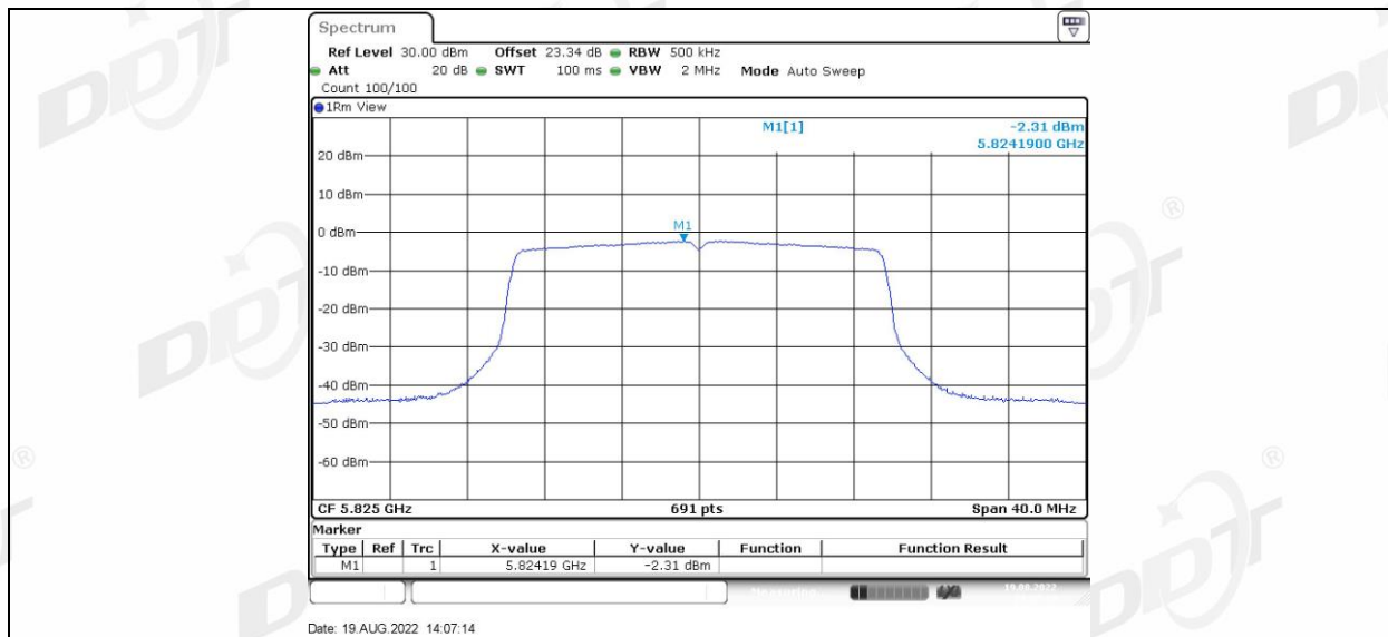
11AX20MIMO_Ant2_5825
