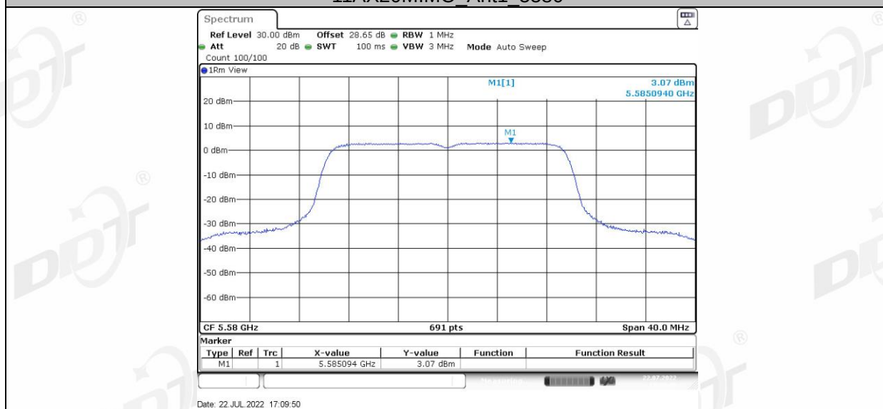
11AX20MIMO_Ant2_5580
