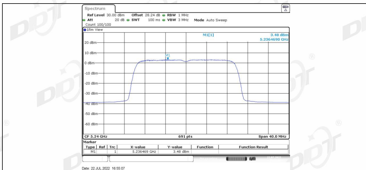
11AX20MIMO_Ant2_5240
