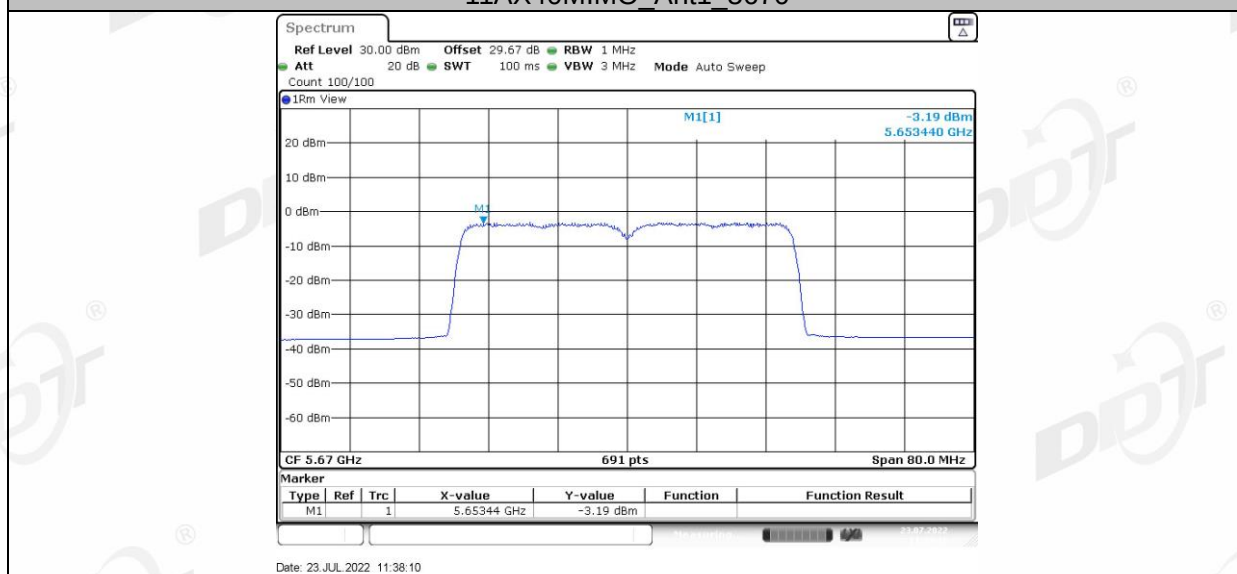
11AX40MIMO_Ant2_5670
