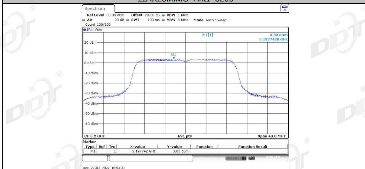
11AX20MIMO_Ant2_5200
