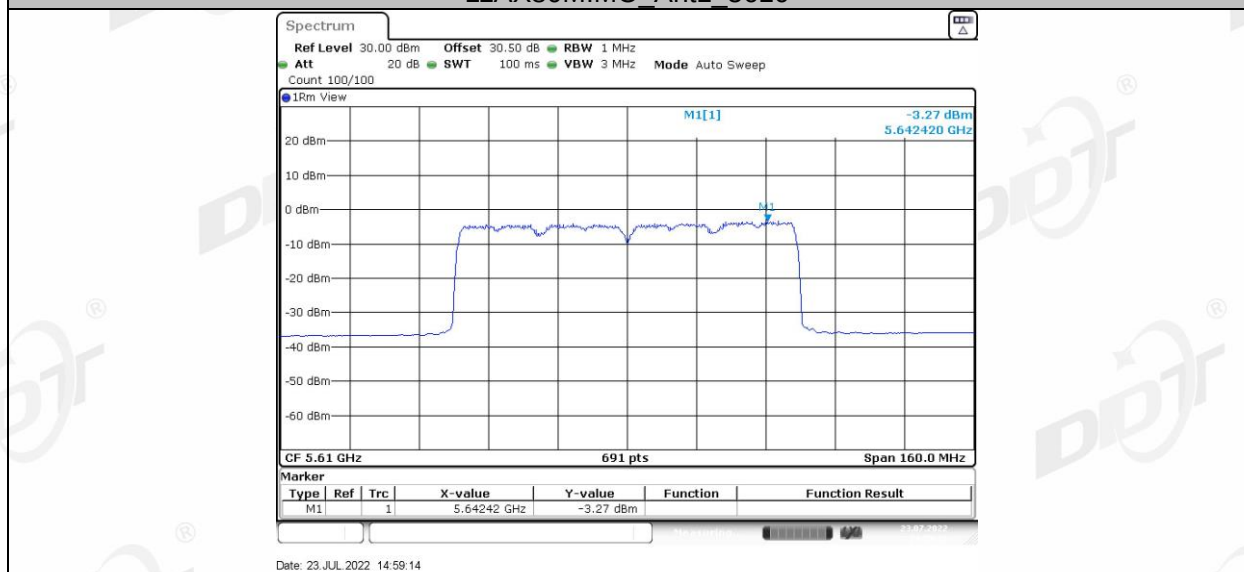
11AX80MIMO_Ant2_5610
