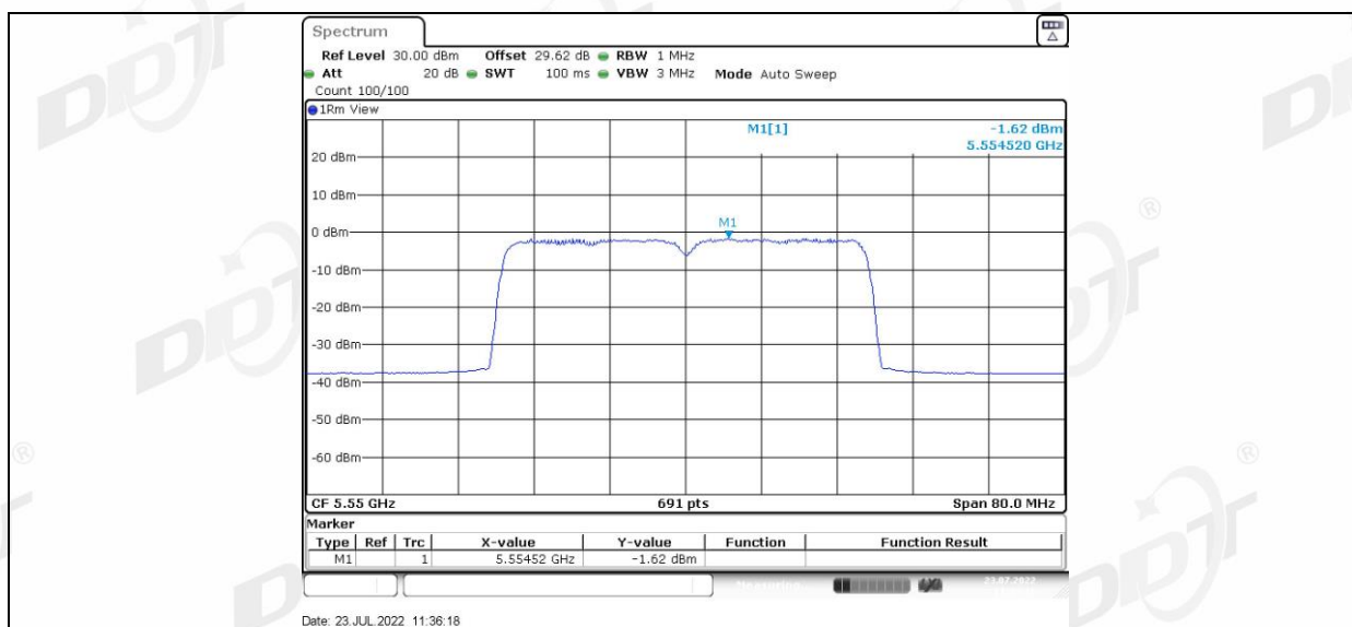
11AX40MIMO_Ant2_5550
