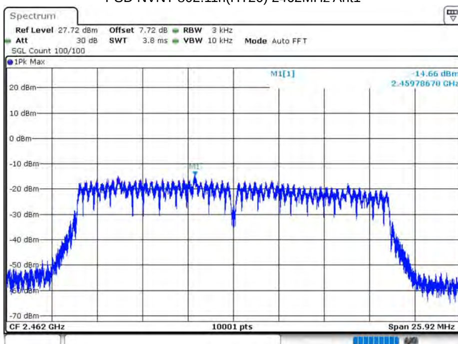
PSD NVNT 802.11n(HT20) 2462MHz Ant1
