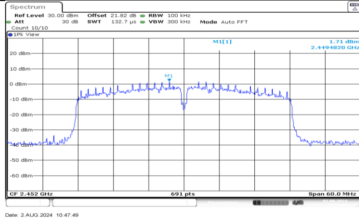
11N40SISO_Ant2_2452_0-Reference
