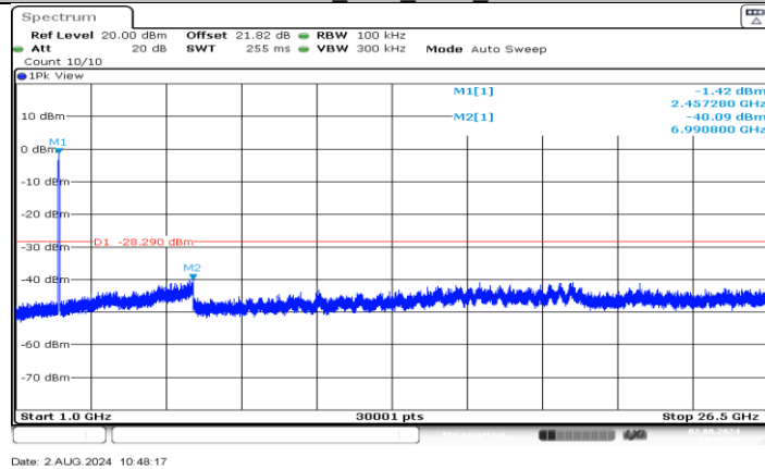
11N40SISO_Ant2_2452_1000-26500
