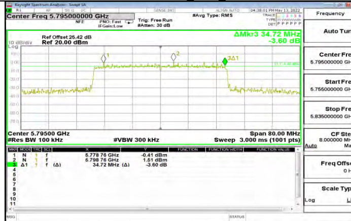
11AX40MIMO Ant1 5795
