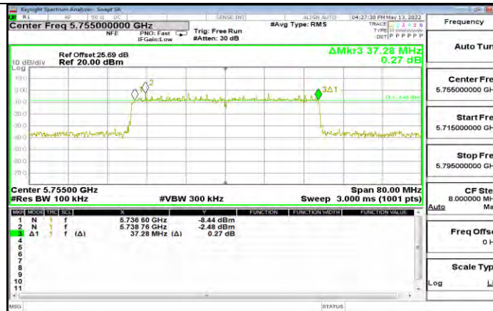
11AX40MIMO Ant1 5755
