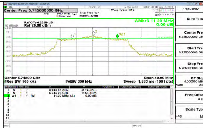
11N20MIMO Ant1 5745
