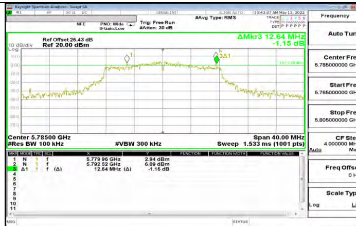
11A_Ant2_5785
