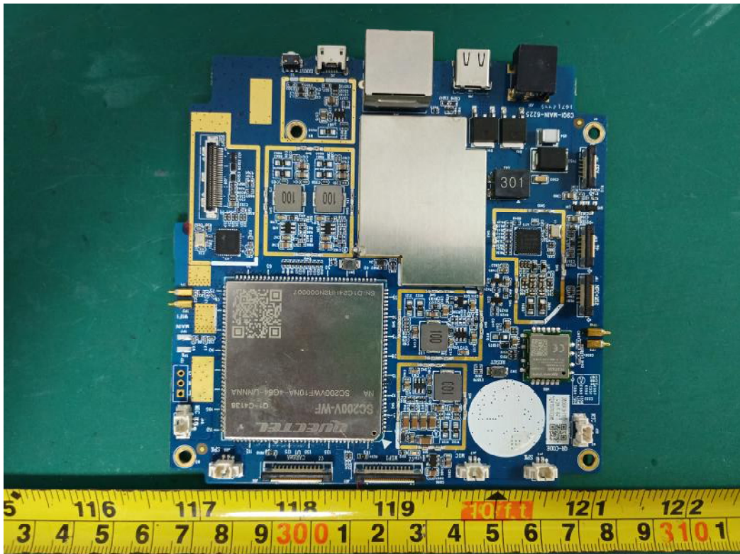
Wi-Fi Module
