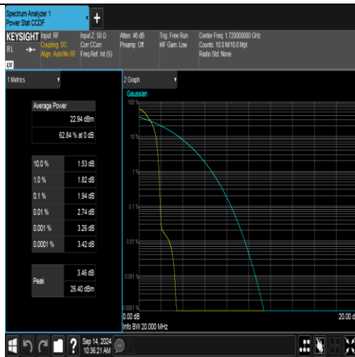
Band66-20MHz-QPSK-132072-1RB#0-PASS
