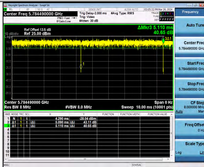
11AX20MIMO_Ant2_5785_52Tone_RU38
