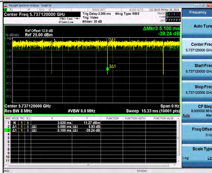
11AX20MIMO_Ant2_5745_52Tone_RU37
