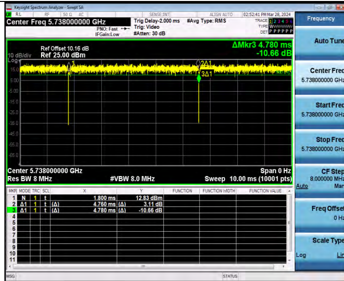
11AX20MIMO_Ant2_5745_26Tone_RU0
