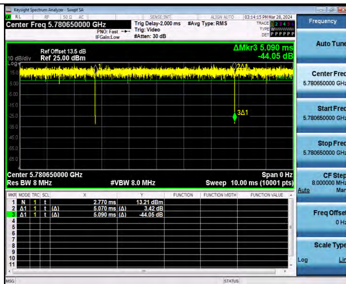
11AX20MIMO_Ant2_5785_106Tone_RU53
