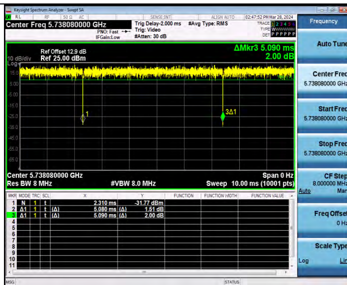
11AX20MIMO_Ant2_5745_106Tone_RU53
