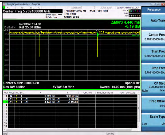
11AX20MIMO_Ant2_5700_52Tone_RU40
