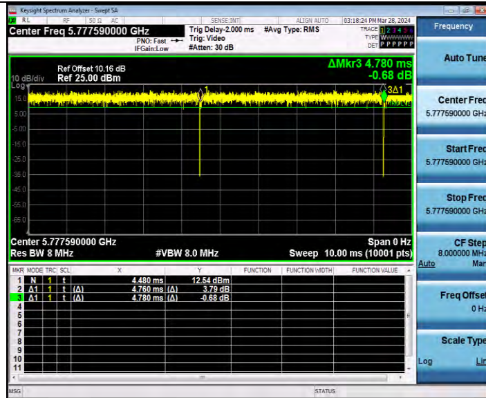
11AX20MIMO_Ant2_5785_26Tone_RU4
