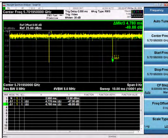
11AX20MIMO_Ant2_5700_26Tone_RU8
