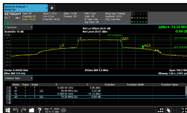
Figure 144 - 802.11ax HE40 SU SP Maximum 99% OBW
