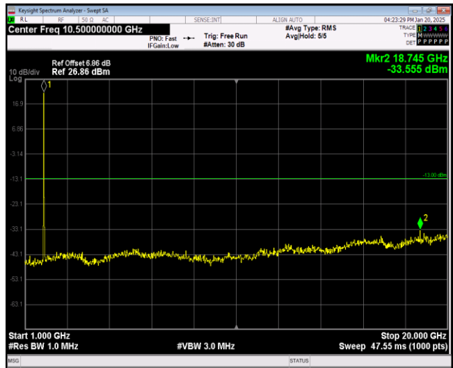
Band2-20MHz-64QAM-18900-1RB#0-Range2:1000~20000MHz
