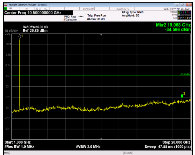
Band2-1.4MHz-QPSK-19193-1RB#0-Range2:1000~2 0000MHz
