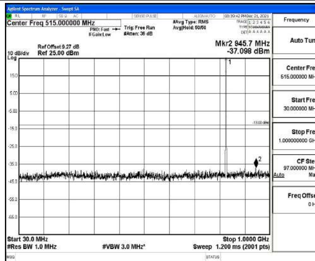
Band26-5MHz-QPSK-26865-1-0-Low-30-1000--37.1-PASS
