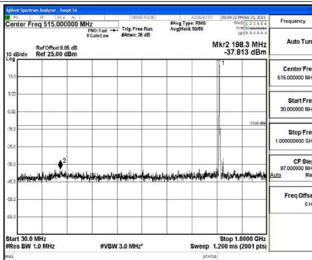
Band26-10MHz-QPSK-26740-1-0-Low-30-1000--37.81-PASS
