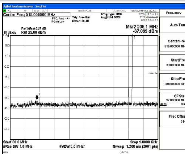
Band26-5MHz-16QAM-26865-1-0-Low-30-1000--37.1-PASS
