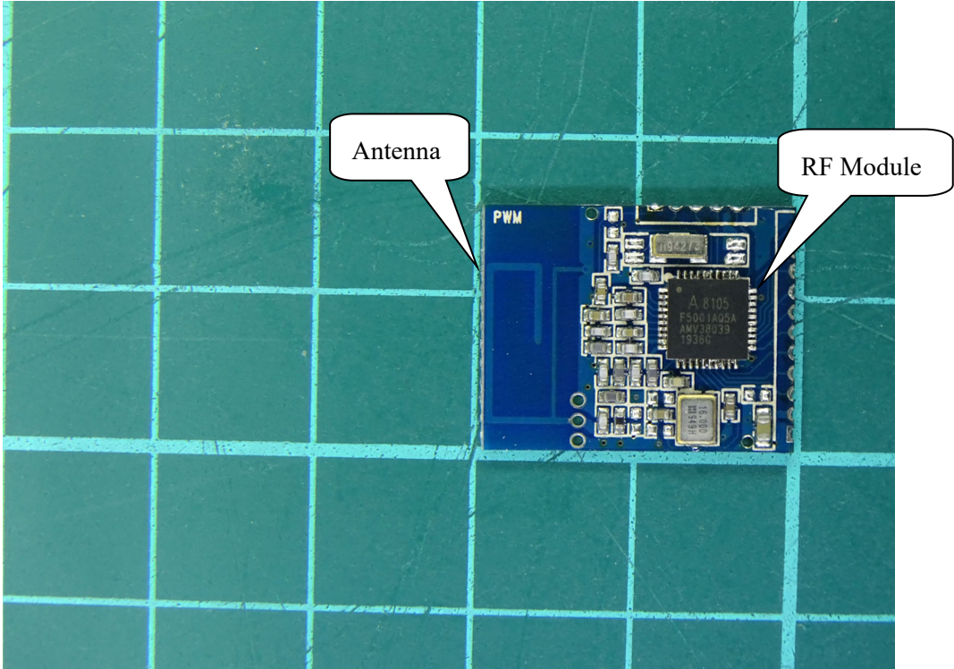
(10) EUT Photo
