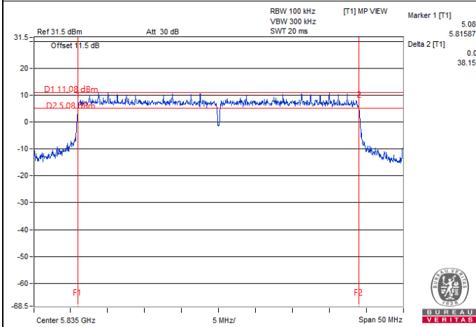
802.11be (EHT40) Beamforming / Chain 3 : CH 167
