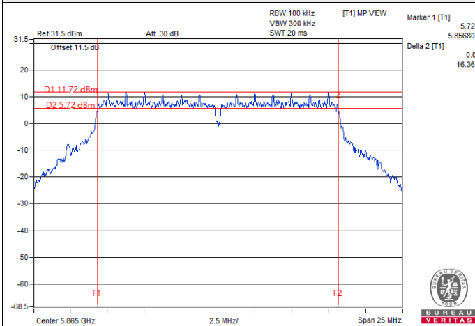
802.11a / Chain 0 : CH 173
