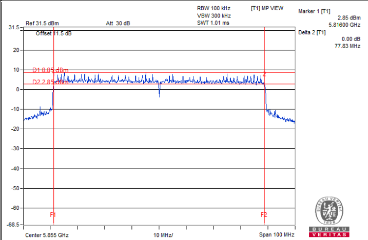
802.11be (EHT80) Beamforming / Chain 3 : CH 171
