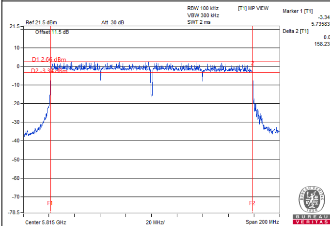
802.11be (EHT160) Beamforming / Chain 3 : CH 163
