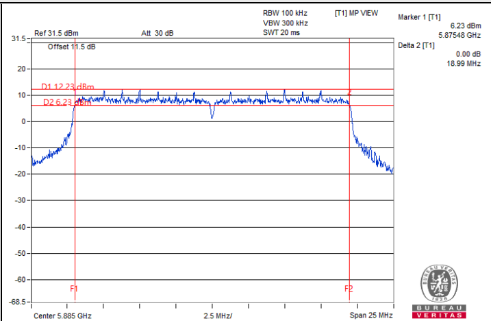
802.11be (EHT20) Beamforming / Chain 3 : CH 177
