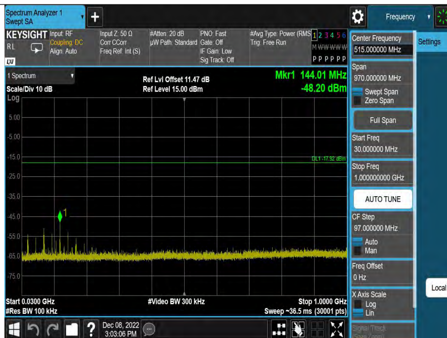
DH5-Ant1-2441-30~1000-2.08
