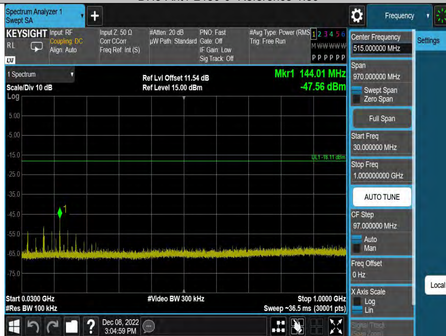
DH5-Ant1-2480-30~1000-1.89
