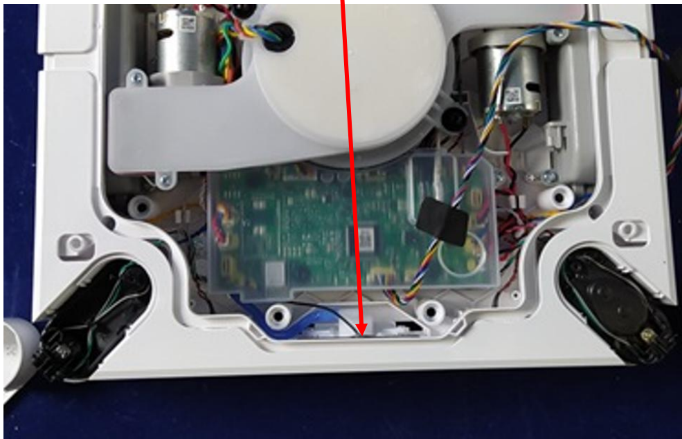
Antenna
