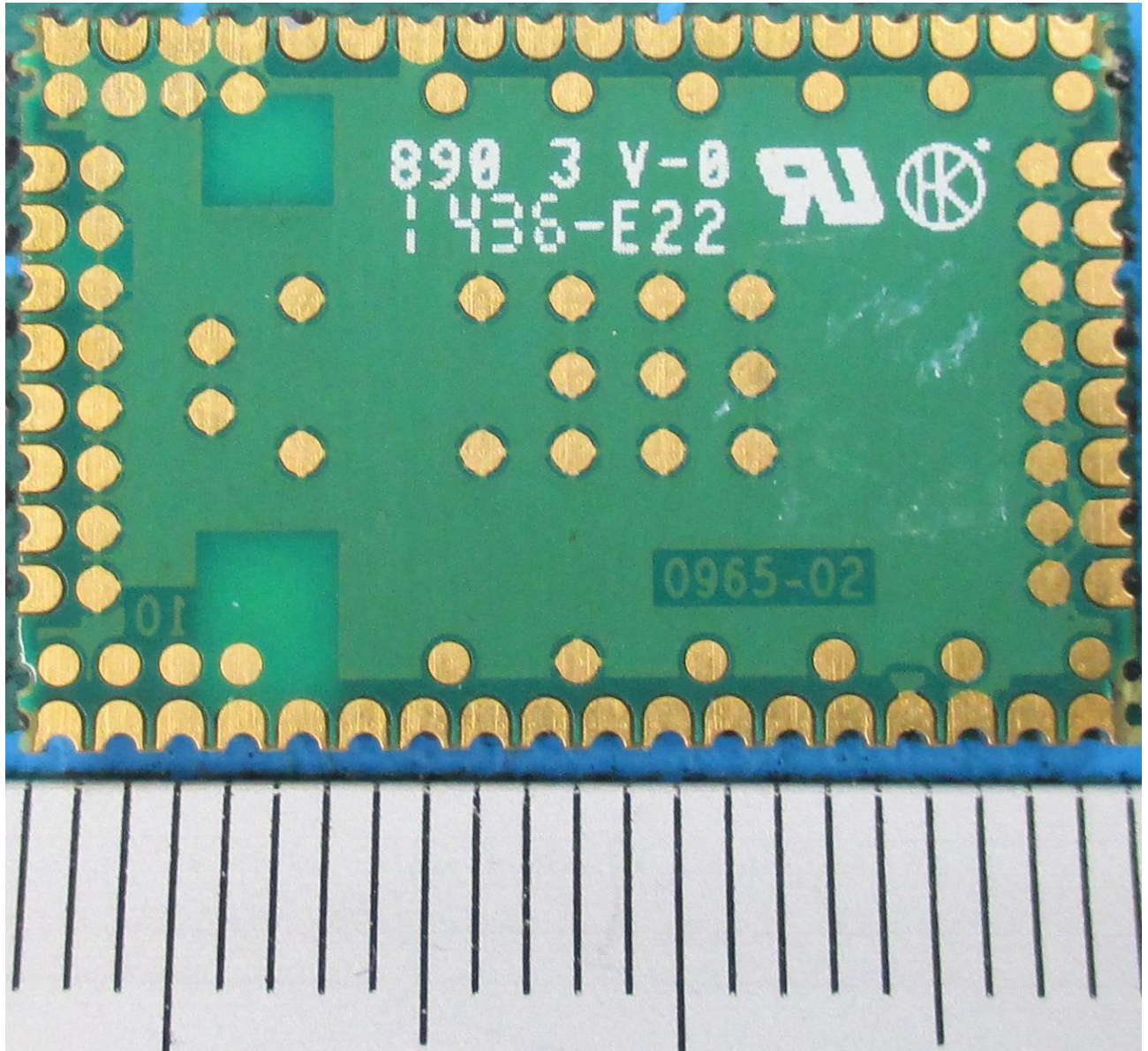
151496_04.jpg: EUT – Bottom View (Odin-W262)
