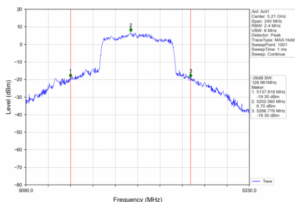
802.11ac (80MHz)
