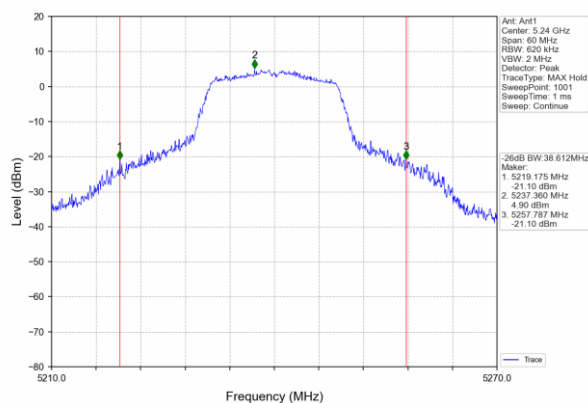
802.11ac (20MHz)
