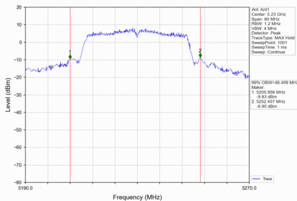
802.11ac (40MHz)
