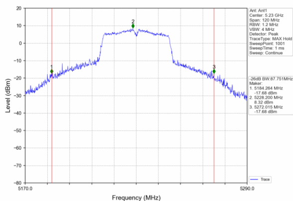
802.11ac (40MHz)
