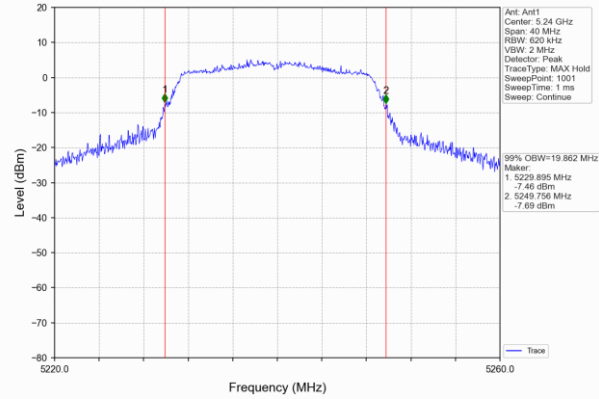
802.11ac (20MHz)
