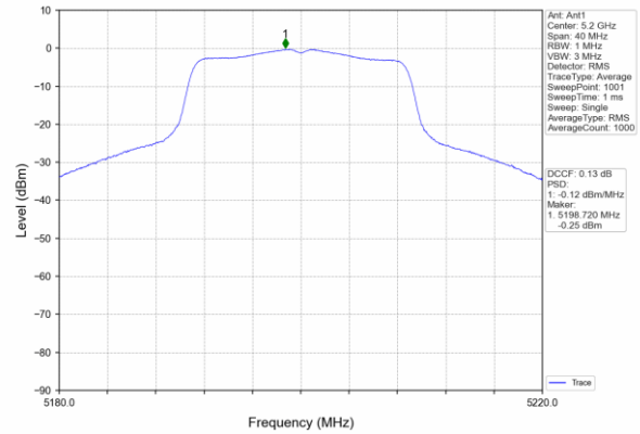
802.11ac (20MHz)
