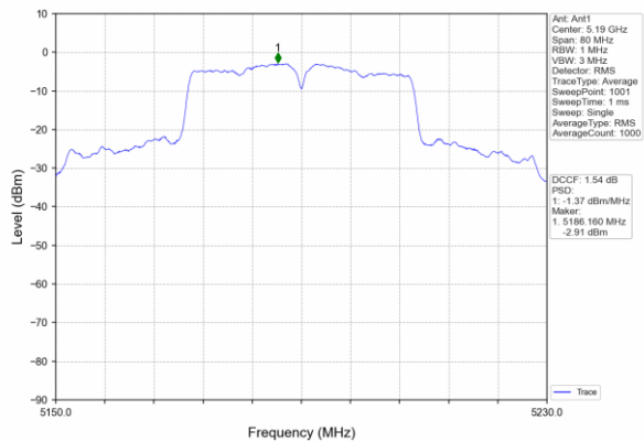
802.11ac (40MHz)
