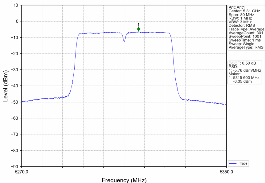
802.11n(HT40)_HCH_5310MHz_Ant1_NTNV
