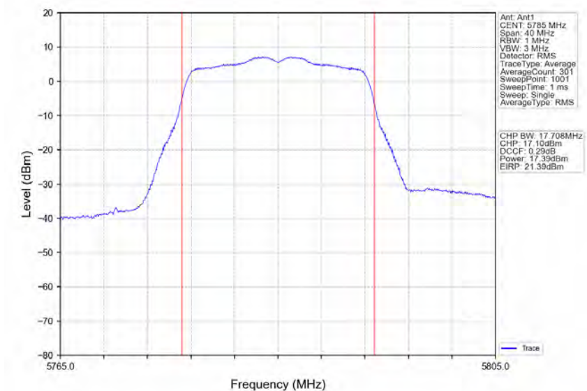
802.11a_MCH_5785MHz_Ant1_NTNV
