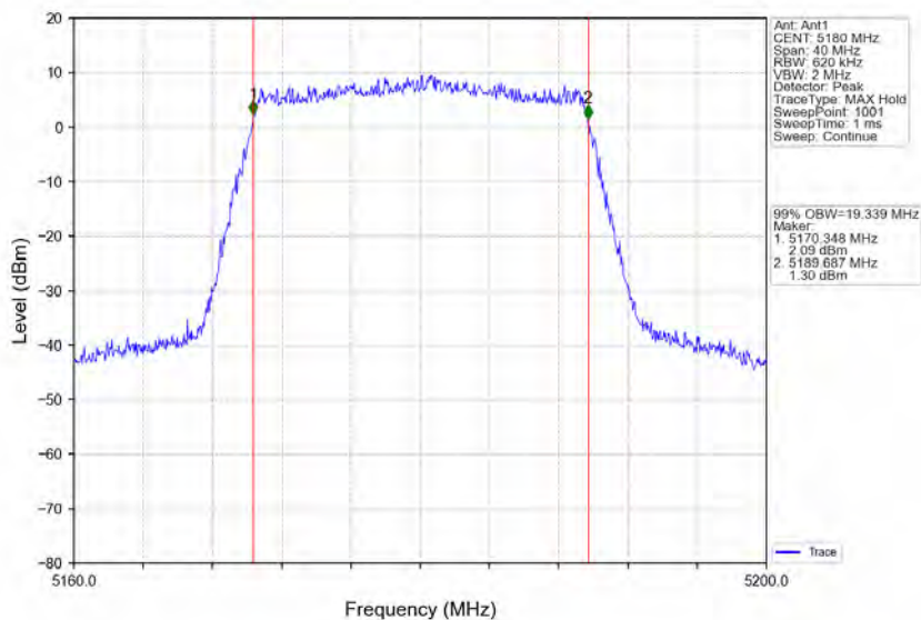
802.11ax(HE20)_LCH_5180MHz_RU242_Ant1_NTNV
