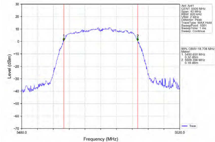
802.11n(HT20)_LCH_5500MHz_Ant1_NTNV
