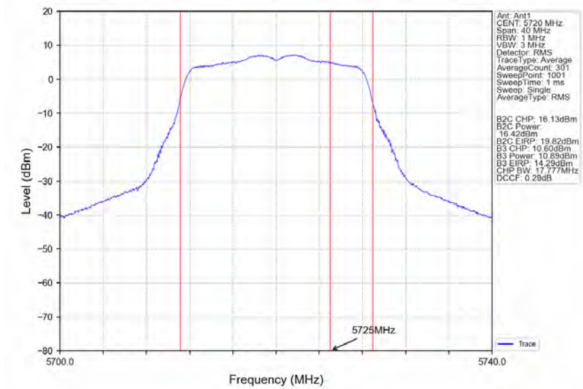
802.11a_HCH_5720MHz_Ant1_NTNV
