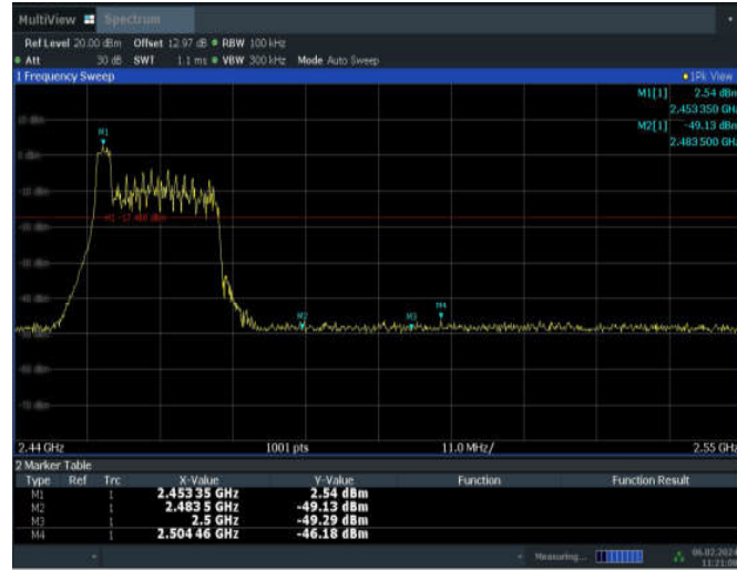
11AX20MIMO_ANT7_High_2462_26Tone_RU8
