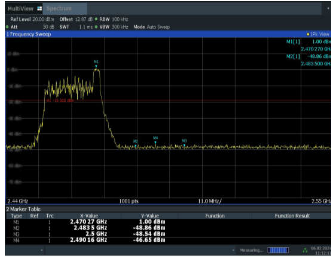
11AX20MIMO_ANT5_High_2462_26Tone_RU8
