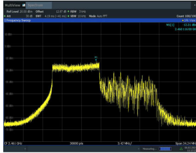
11AX20MIMO_ANT5_2462_106Tone_RU53
