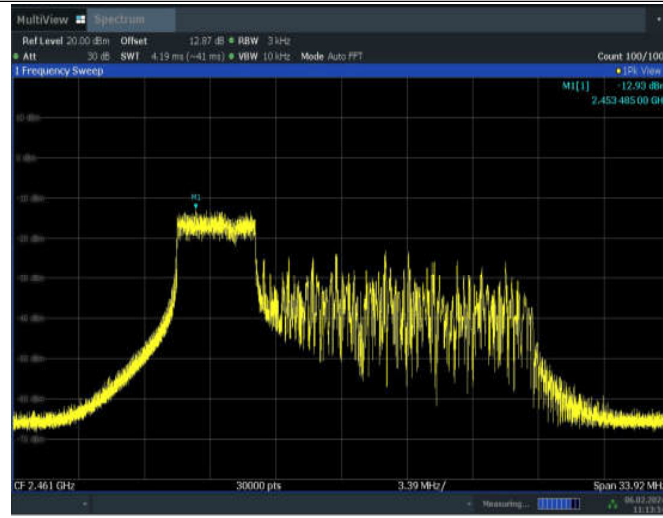
11AX20MIMO_ANT5_2462_52Tone_RU37
