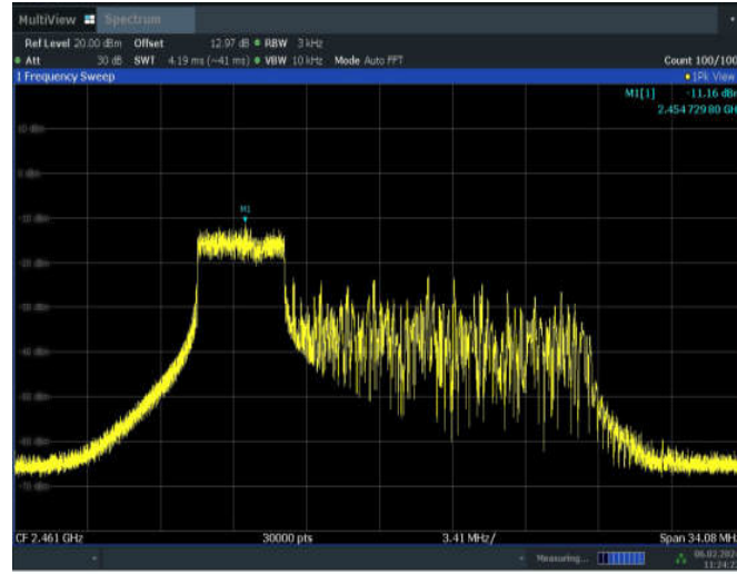
11AX20MIMO_ANT7_2462_52Tone_RU37
