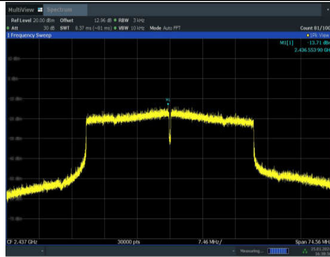
11AX40MIMO_ANT7_2437
