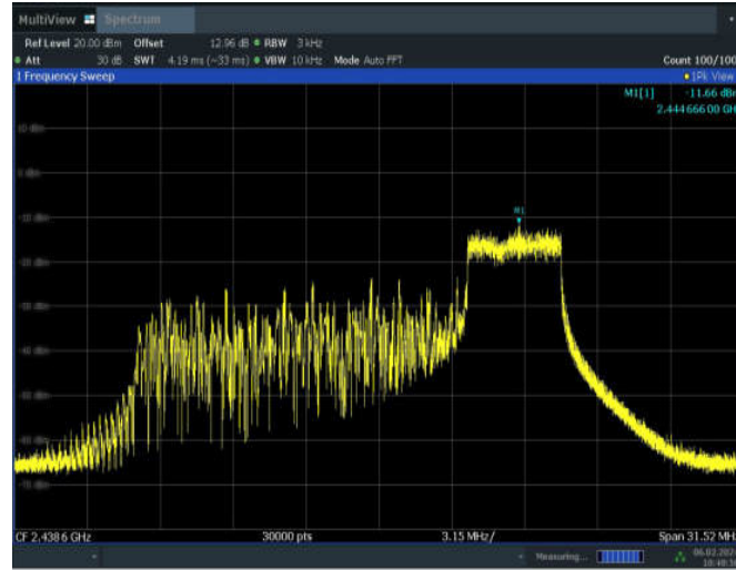
11AX20MIMO_ANT5_2437_106Tone_RU53
