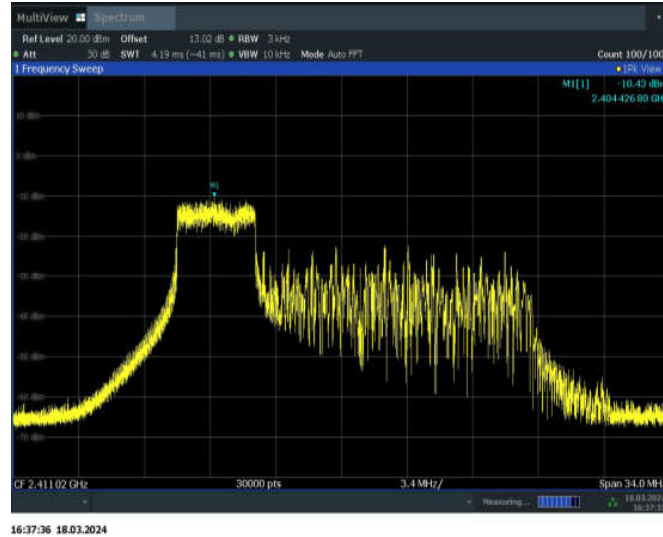
11AX20MIMO_ANT5_2412_52Tone_RU40
