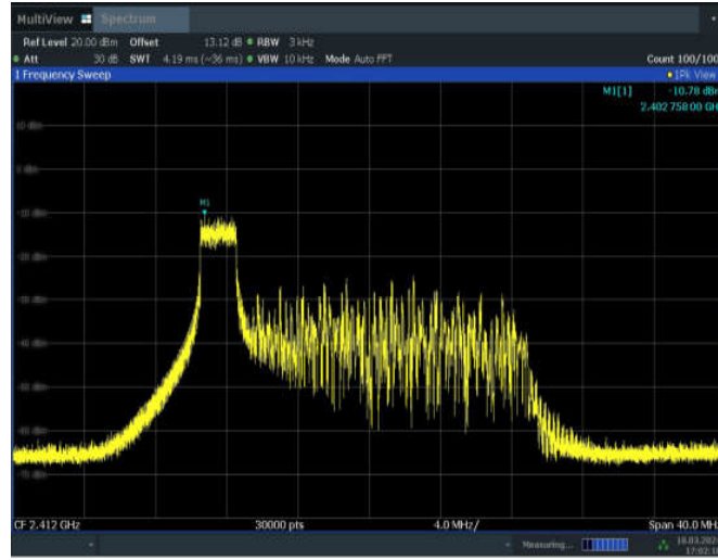
11AX20MIMO_ANT7_2412_26Tone_RU0
