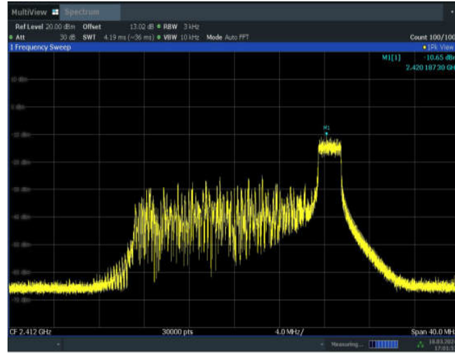
11AX20MIMO_ANT5_2412_52Tone_RU37
