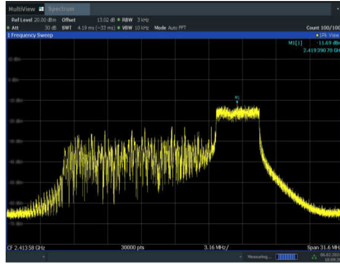
11AX20MIMO_ANT5_2412_106Tone_RU53
