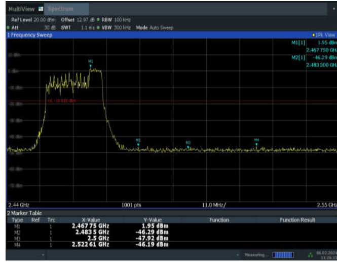
11AX20MIMO_ANT7_High_2462_52Tone_RU40
