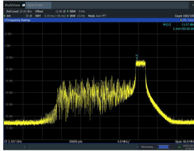
11AX20MIMO_ANT5_2437_52Tone_RU37
