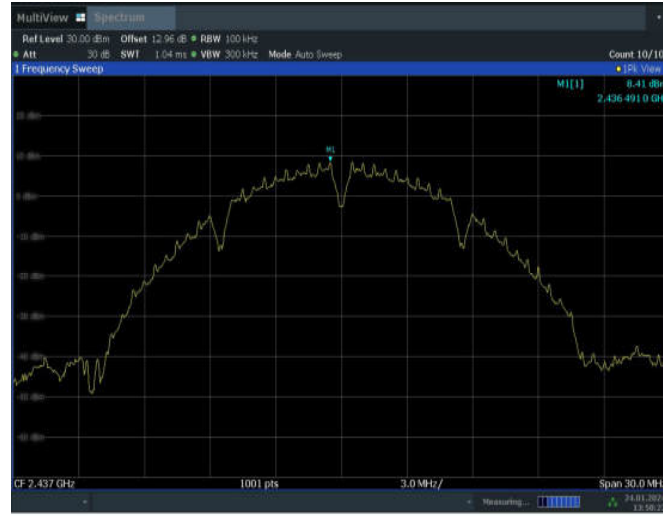
11B_ANT5_2437_0~Reference
