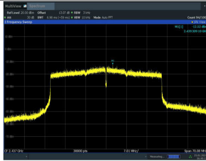
11AX40MIMO_ANT7_2437
