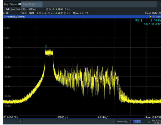
11AX20MIMO_ANT5_2437_26Tone_RU0
