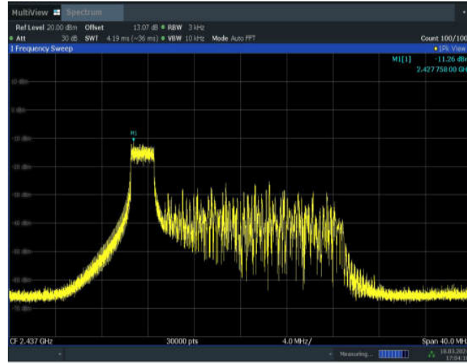
11AX20MIMO_ANT7_2437_26Tone_RU0
