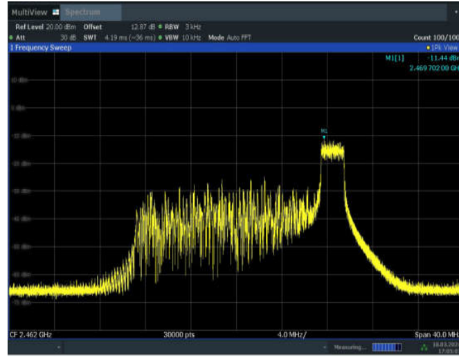
11AX20MIMO_ANT5_2462_52Tone_RU37
