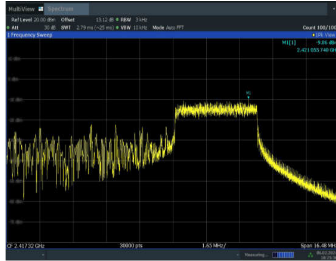
11AX20MIMO_ANT7_2412_106Tone_RU53
