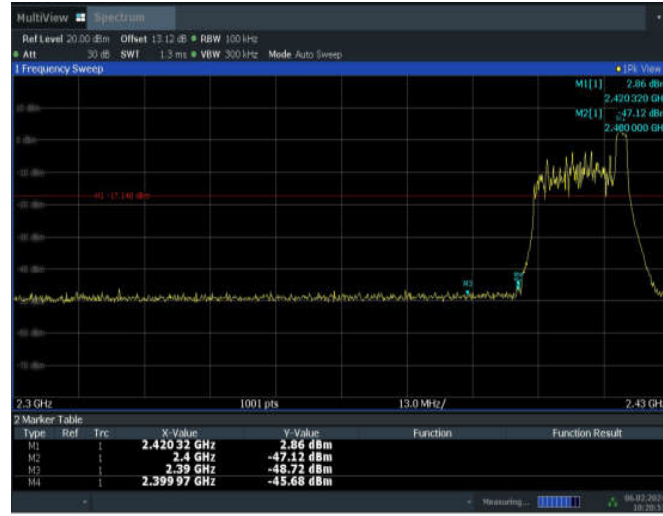
11AX20MIMO_ANT7_Low_2412_26Tone_RU8
