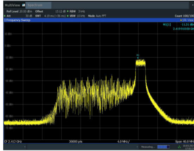
11AX20MIMO_ANT7_2412_52Tone_RU37
