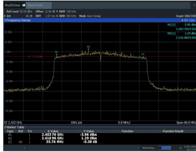
11AX40SISO_ANT5_2422
