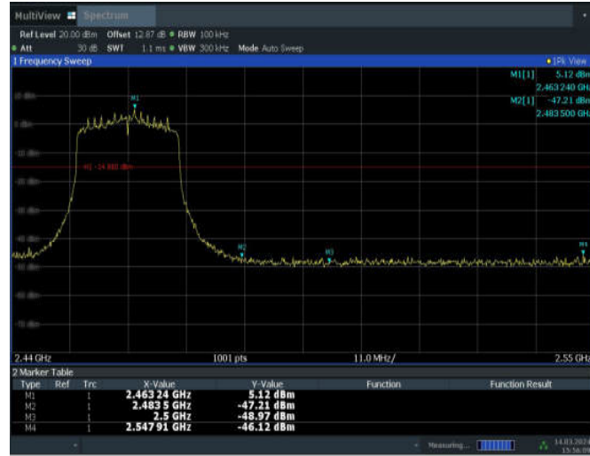
11AX20MIMO_ANT7_High_2462
