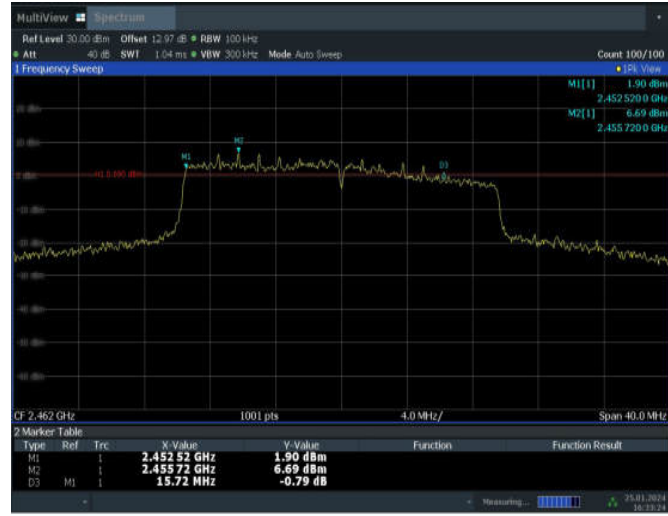
11AX20MIMO_ANT7_2462
