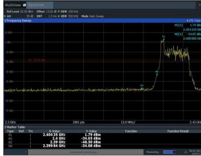
11AX20MIMO_ANT5_Low_2412_26Tone_RU0
