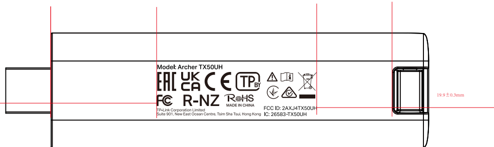
尺寸图(垂直方向上目视居中)
