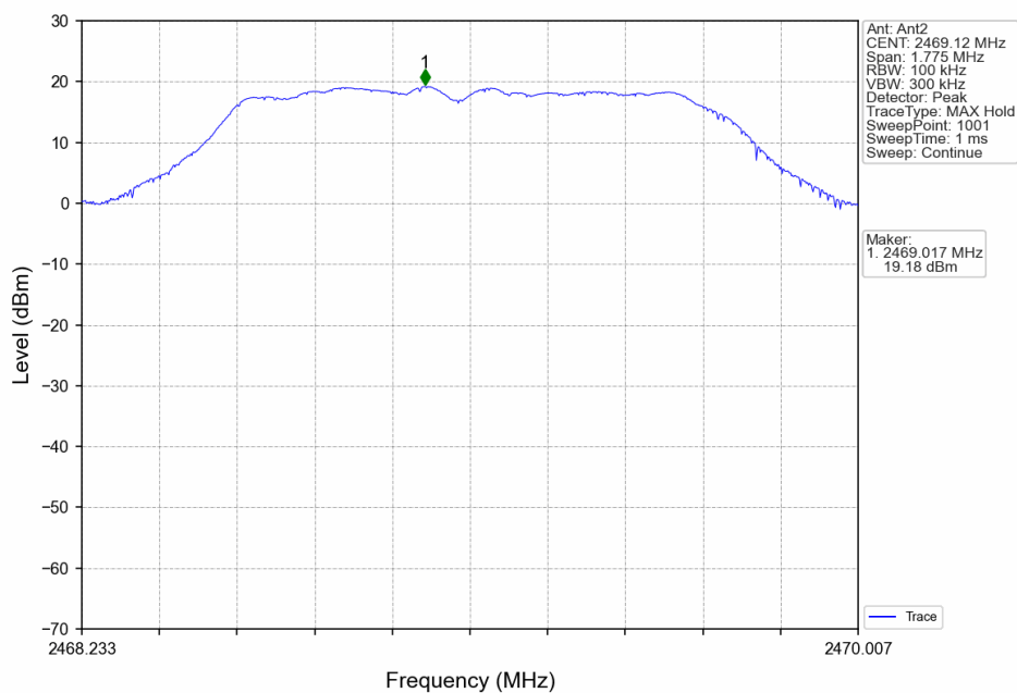
1.4M_HCH_2469.12MHz_Ant2_NTNV
