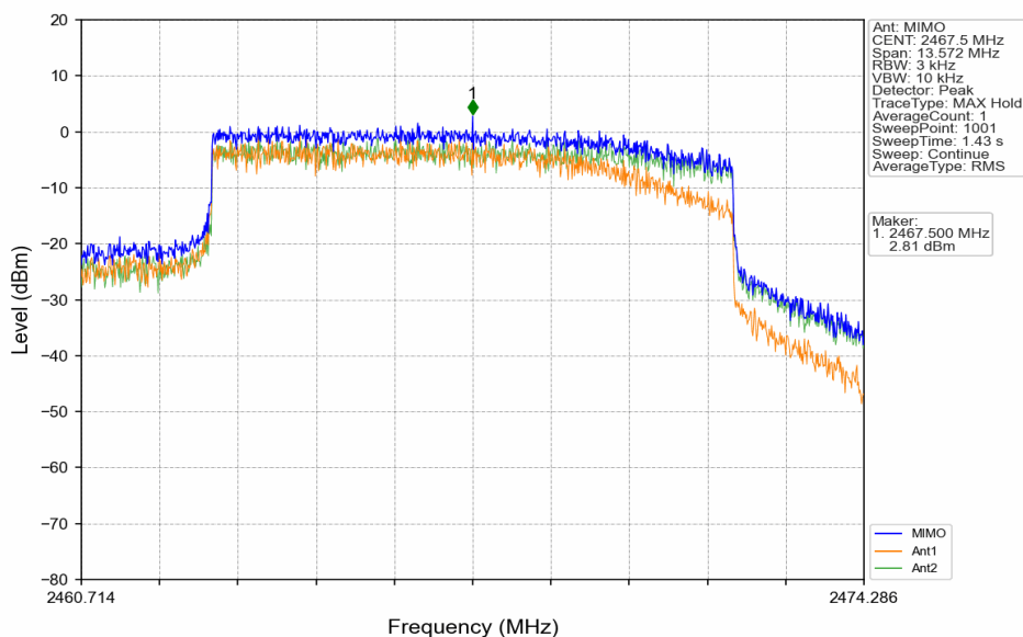
10M_HCH_2467.5MHz_MIMO_NTNV
