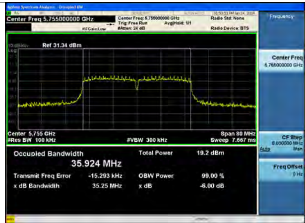
802.11ac(VHT40) (CH 151)
