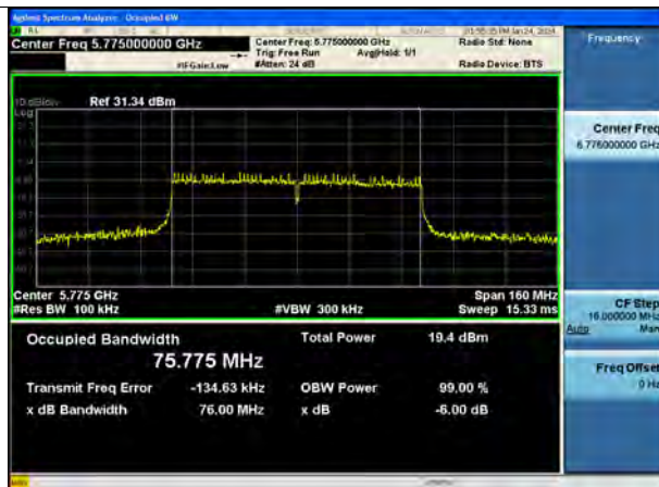
802.11ac(VHT80) (CH 155)
