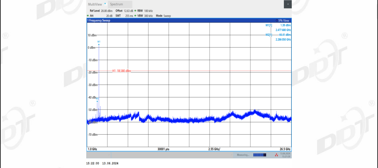
BLE_2M_Right side_2478_1000~26500
