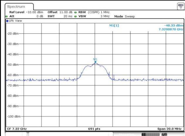
7320MHz - PK
