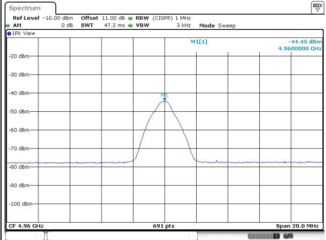
4960MHz - AV
