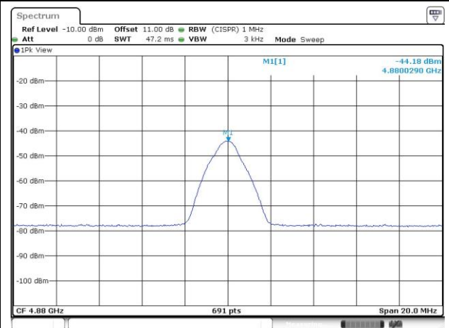
4880MHz - AV
