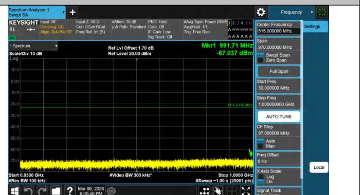
Band25-20MHz-QPSK-26365-1RB#99-30~1000-PASS
