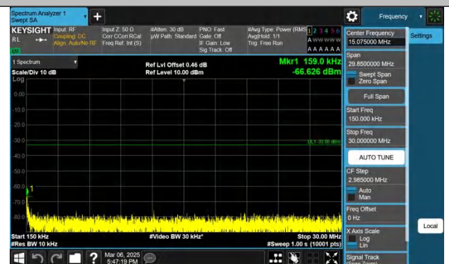
Band25-10MHz-QPSK-26365-1RB#0-0.15~30-PASS
