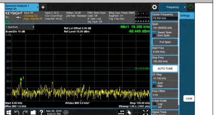
Band25-20MHz-QPSK-26365-1RB#99-0.009~0.15-PASS
