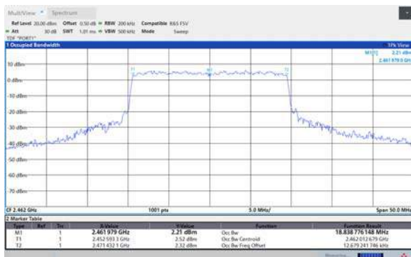
RU 242T offset 61 / 2 462 MHz
